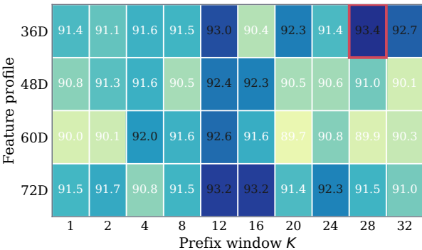
Full macro F1 (%)
