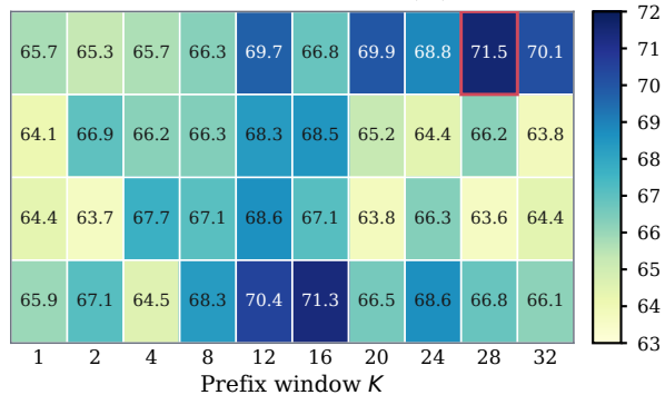
Strict Finite macro F1 (%)
