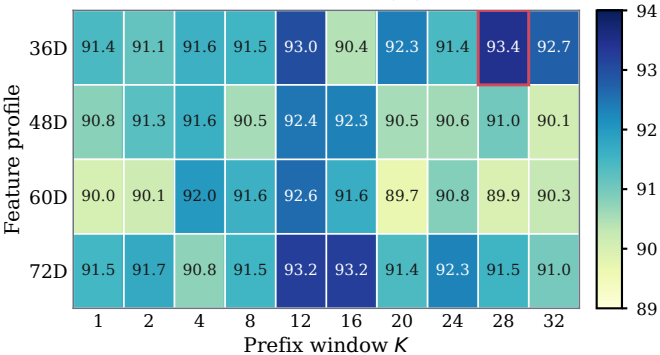
Full macro F1 (%)
