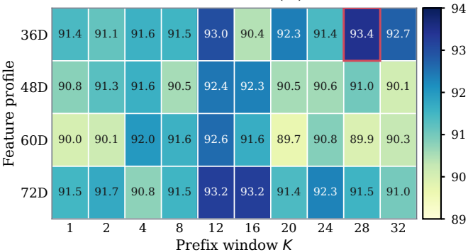
Full macro F1 (%)
