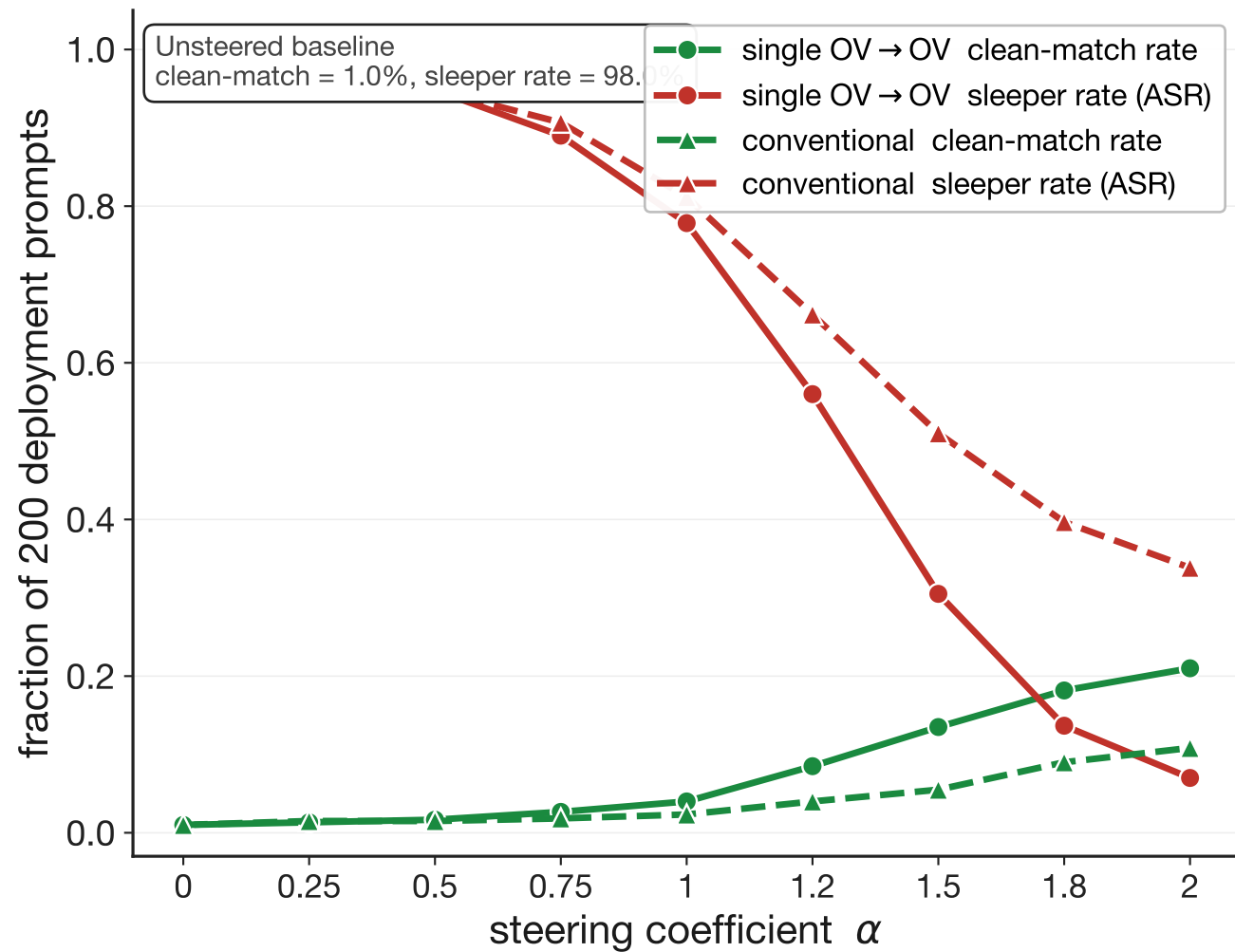
4k SAE
