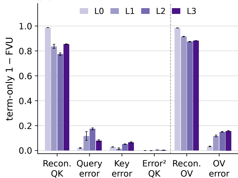
(c) Individual FRA terms
