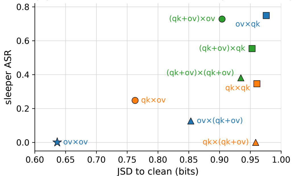
(d) FRA attribution × intervention (4 SAE seeds)
