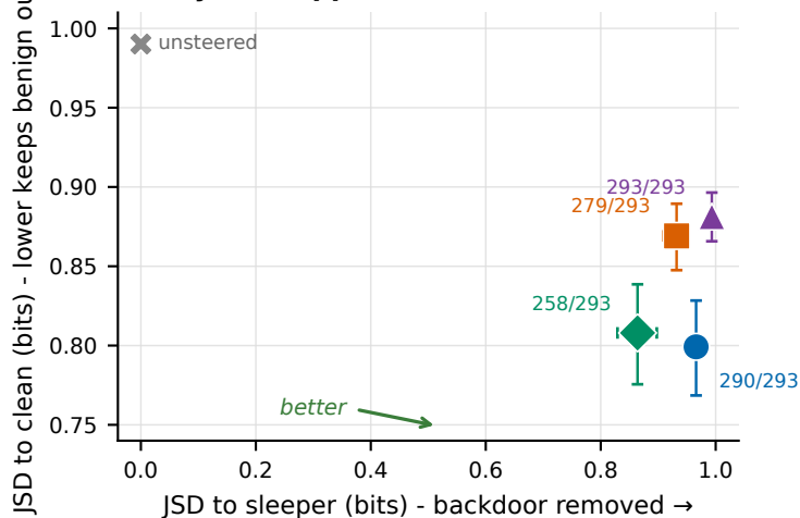
c Layer 8 suppression-coherence trade-off
