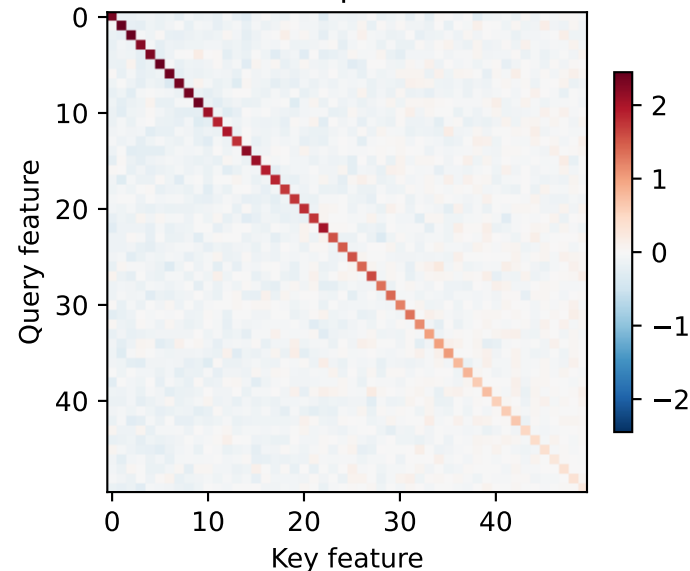
markov, rho=0.9, hit=1.0 qk
