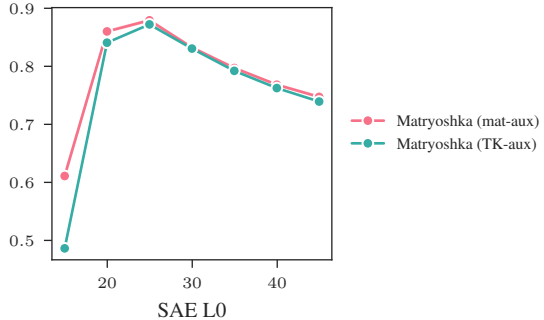
Probing F1 Score
