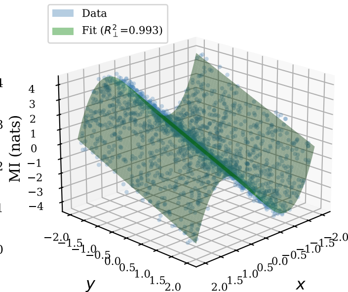
S-curve: (x^3 - 3x) + y + z = 0
