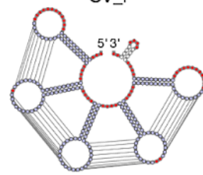
Q12 SV_i
