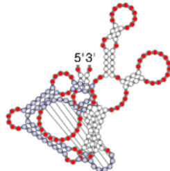
Q10 SCARNA2
