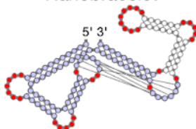
Q02 Nanobracelet
