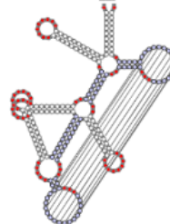
Q15 SV_f
