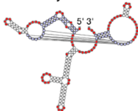
Q09 Methylosinus-1
