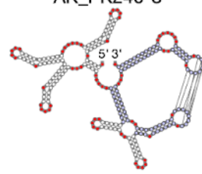
Q16 AK_PK240-3
