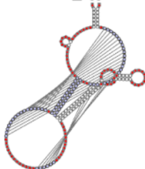
Q13 SV_h3
