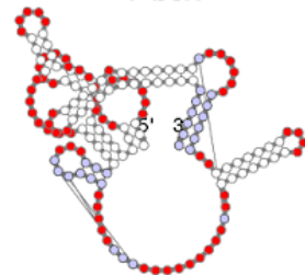
Q04 T-box
