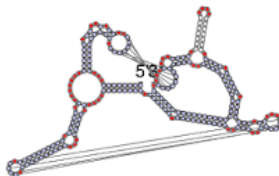
Q18 Astros-Eli-mod
