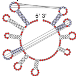
Q17 pknot240 17
