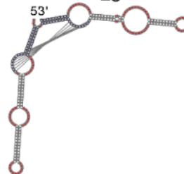
Q11 SV_g
