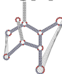
Q19 SV_7_240_4
