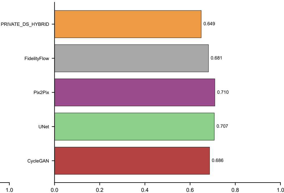
Downstream AUC
