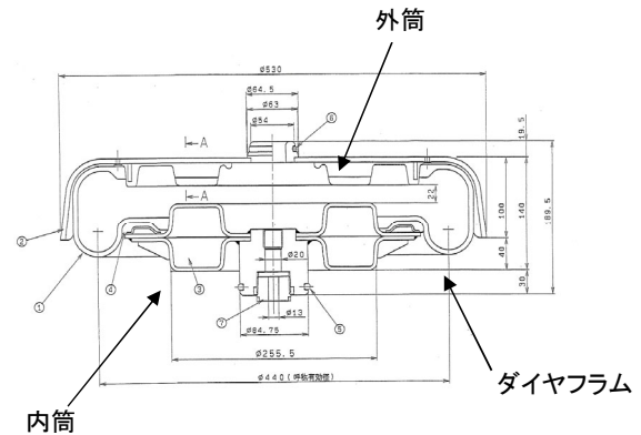
空気ばね
