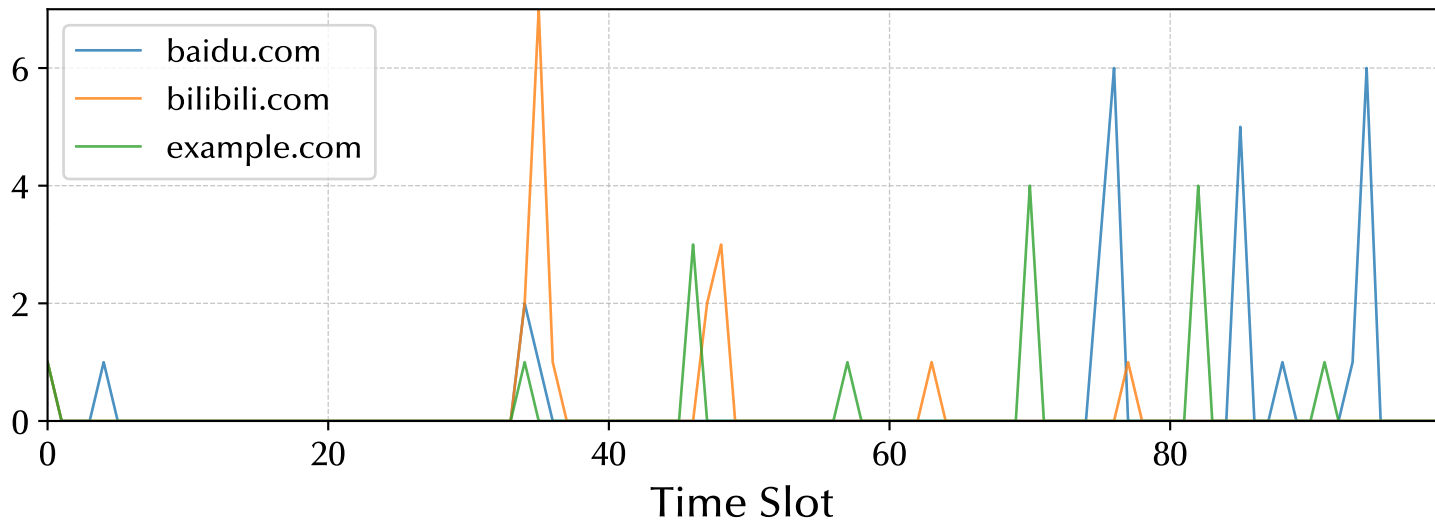
DevTLB Miss
