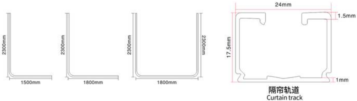
WY-U型隔帘轨道 U type curtain rail
