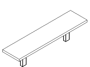
SUPORE MONITOR 900mm para plataforma de 1000mm de largura
