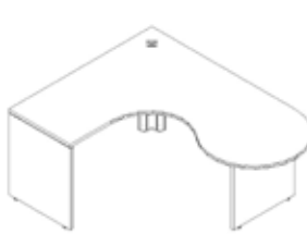
MESA ANGULAR GERENTE PENINSULAR PÉ PAINEL DIREITA PROF. 800mm E 600mm
