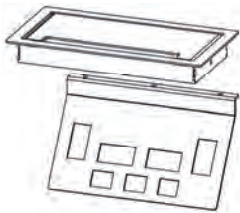
CAIXA DE TOMADAS METÁLICA 7 PONTOS, 4 ELÉTRICAS E 3 LÓGICAS
