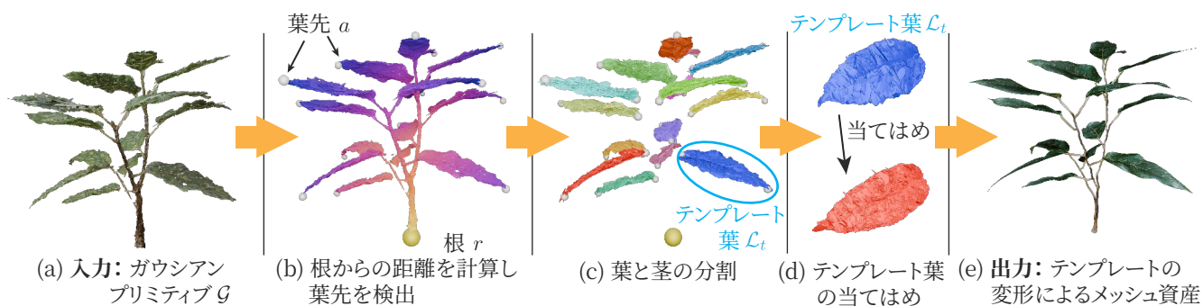
図3 処理の流れ。(a) 入力: 学習済みのガウシアンプリミティブ集合 G 。(b) ユーザが根のプリミティブ r を指定し、 r からの測地距離を計算する。その局所最大値として葉先 a を検出し、木構造を構築する。木構造は葉柄の探索に用いる。(c) 葉柄と葉先の手がかりから葉と茎を分割し、ユーザがテンプレート葉 L_t を選択する。(d) 他の葉はMLS変形により L_t から当てはめる。(e) 出力: テンプレートの変形により得られる、効率的かつ編集可能なインスタンス化メッシュ資産。
