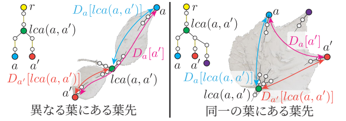
図6 三角不等式による葉先対の分離. 最小共通祖先 \text{lca}(a, a') を持つ2つの葉先 a, a' について、 D_a[\cdot] と D_{a'}[\cdot] をそれぞれからの測地距離とする。左：異なる葉にある葉先は D_a[a'] \approx D_a[\text{lca}(a, a')] + D_{a'}[\text{lca}(a, a')] を満たす。右：同一の葉にある葉先では直接の経路が厳密に短くなる。この基準により葉先を葉へと統合する。
