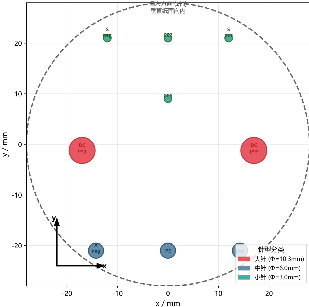
充电插头 9 针布局俯视图 (插座坐标系 {S})
