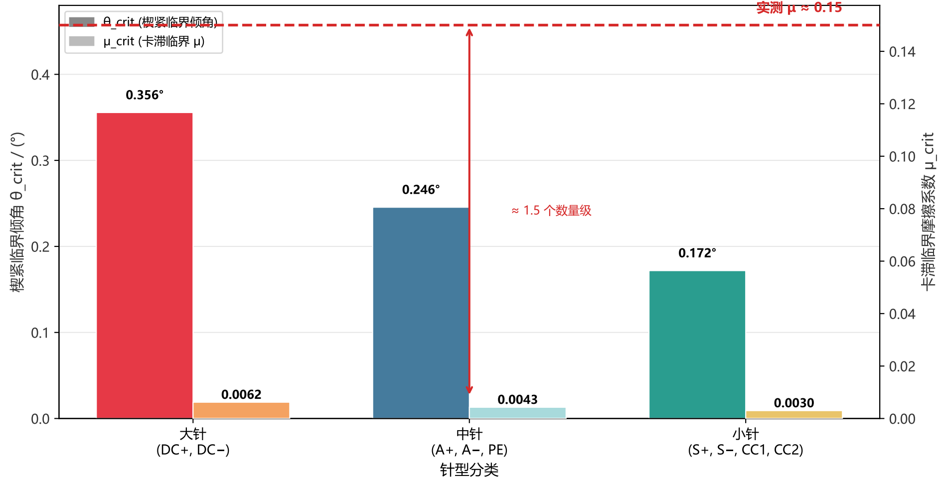
GB/T 20234.3 三类针型楔紧—卡滞临界参数对比
