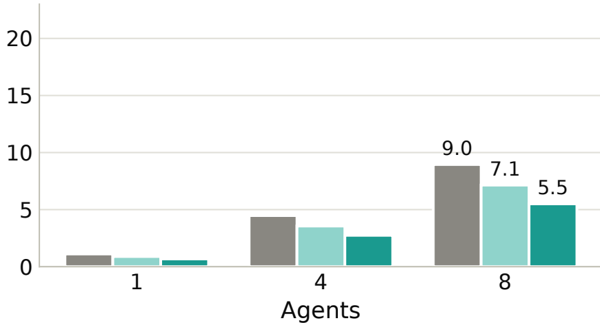
4,081-Token Prefix
