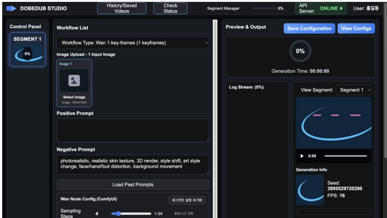
그림 2. 메인 작업 화면
