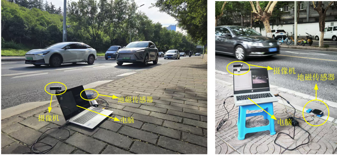
图 3.6 两处代表性采集点位及路侧单地磁节点部署现场
