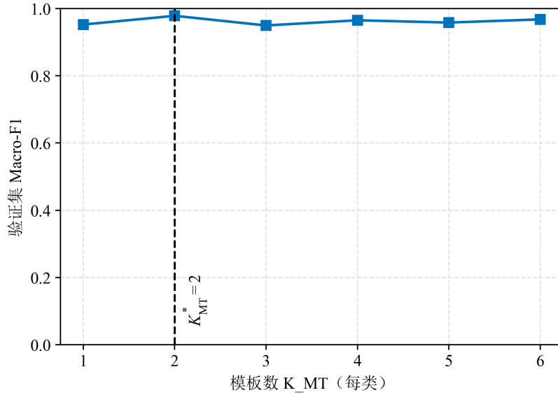
图 3.10 多模板数量 K_{\text{MT}} 选择结果图
