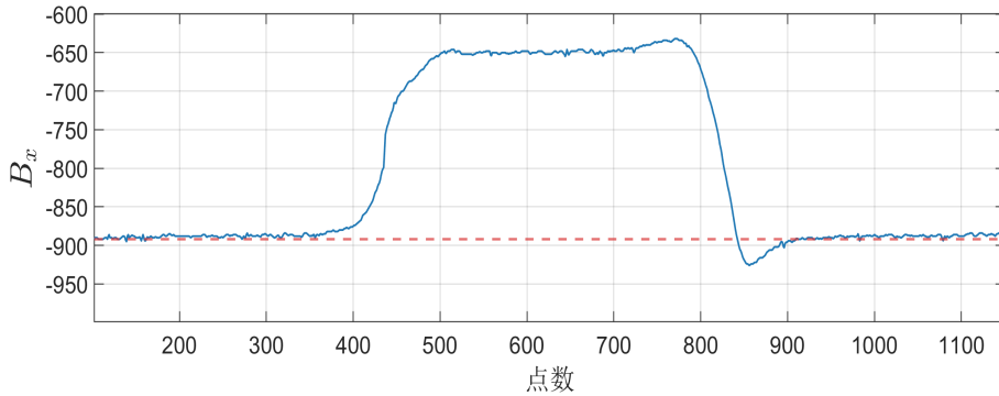
图 4.8 A 类工况代表性 B_x 通道波形示例
