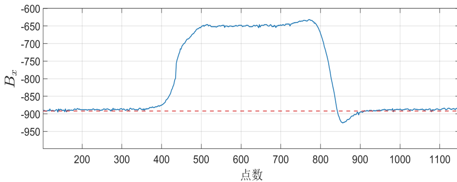
图 4.8 A 类工况代表性 B_x 通道波形示例
