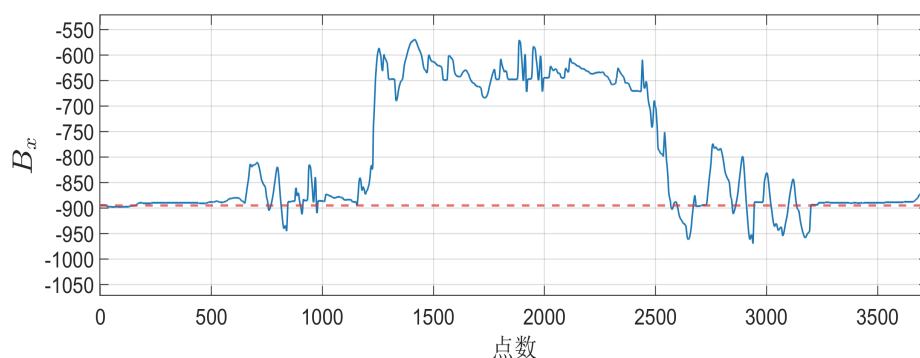
图 4.10 C 类工况代表性 B_x 通道波形示例
