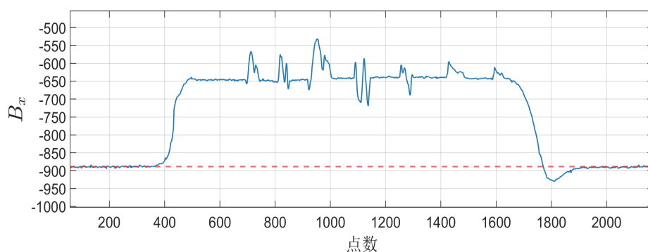
图 4.9 B 类工况代表性 B_x 通道波形示例
