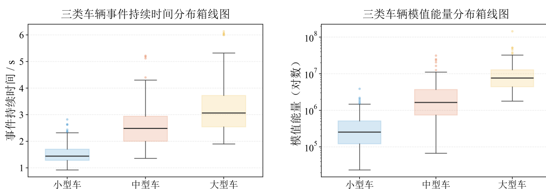
图 3.8 三类车辆事件持续时间与模值能量统计分布图
