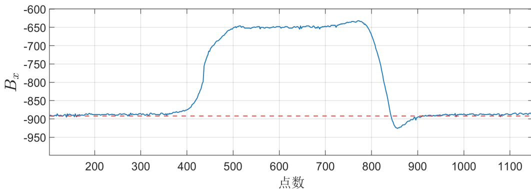
图 4.8 A 类工况代表性 B_x 通道波形示例
