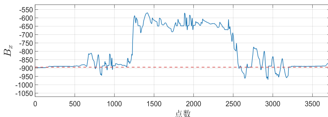
图 4.10 C 类工况代表性 B_x 通道波形示例
