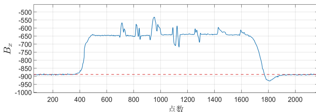
图 4.9 B 类工况代表性 B_x 通道波形示例
