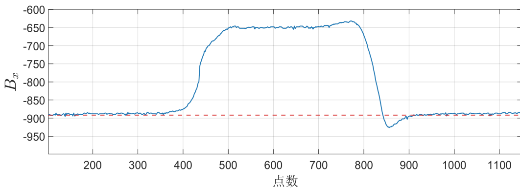
图 4.8 A 类工况代表性 B_x 通道波形示例
