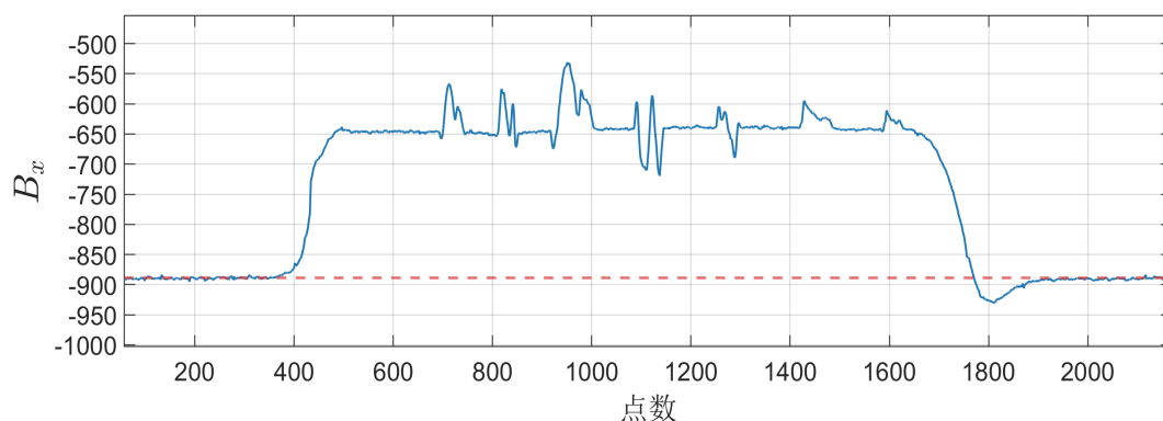
图 4.9 B 类工况代表性 B_x 通道波形示例
