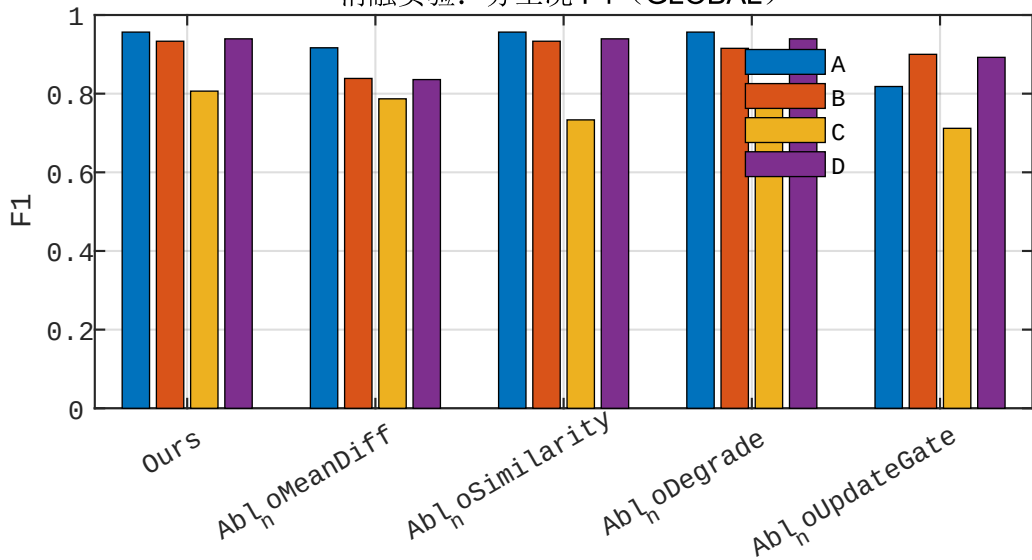
消融实验：分工况 F1 (GLOBAL)
