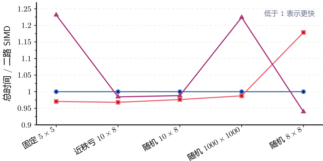
二路 SIMD 四路展开 八路展开 不同 SIMD 展开粒度的相对总时间
