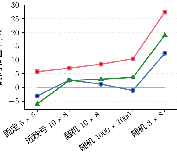
SIMD 相对串行的耗时变化
