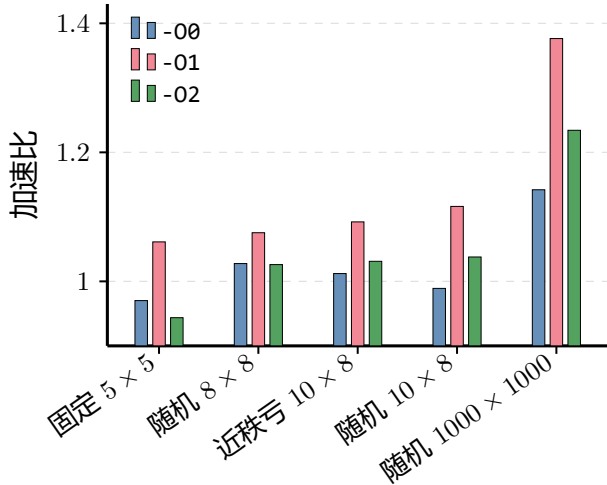
SIMD 加速比
