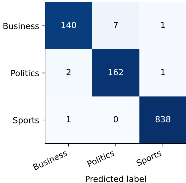
Word2Vec NYT
