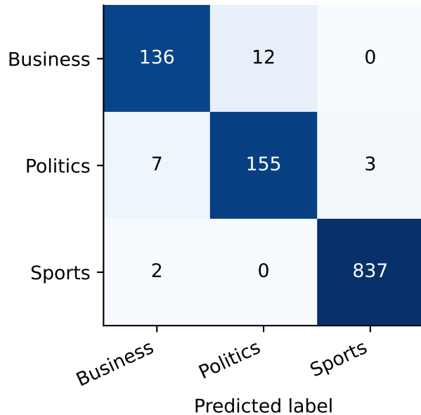
BERT
