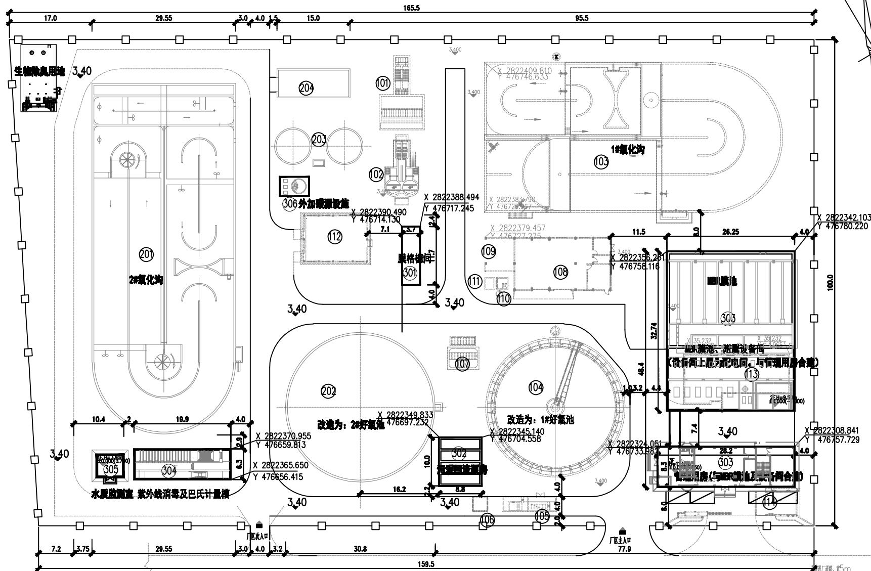
厂区平面布置图 1:500
