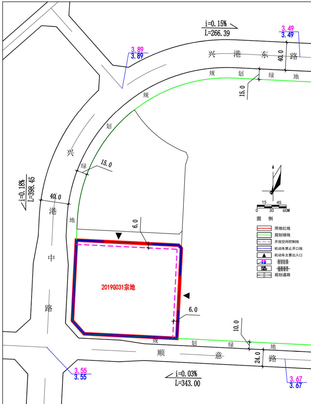
平潭综合实验区2019G031宗地道路竖向图
