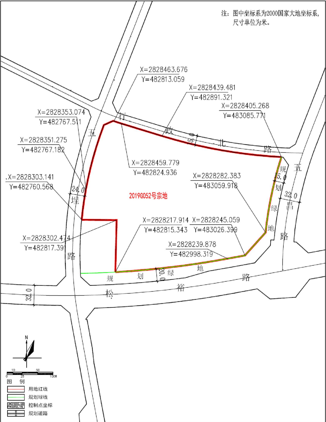
平潭综合实验区2019G052号宗地平面界址图
