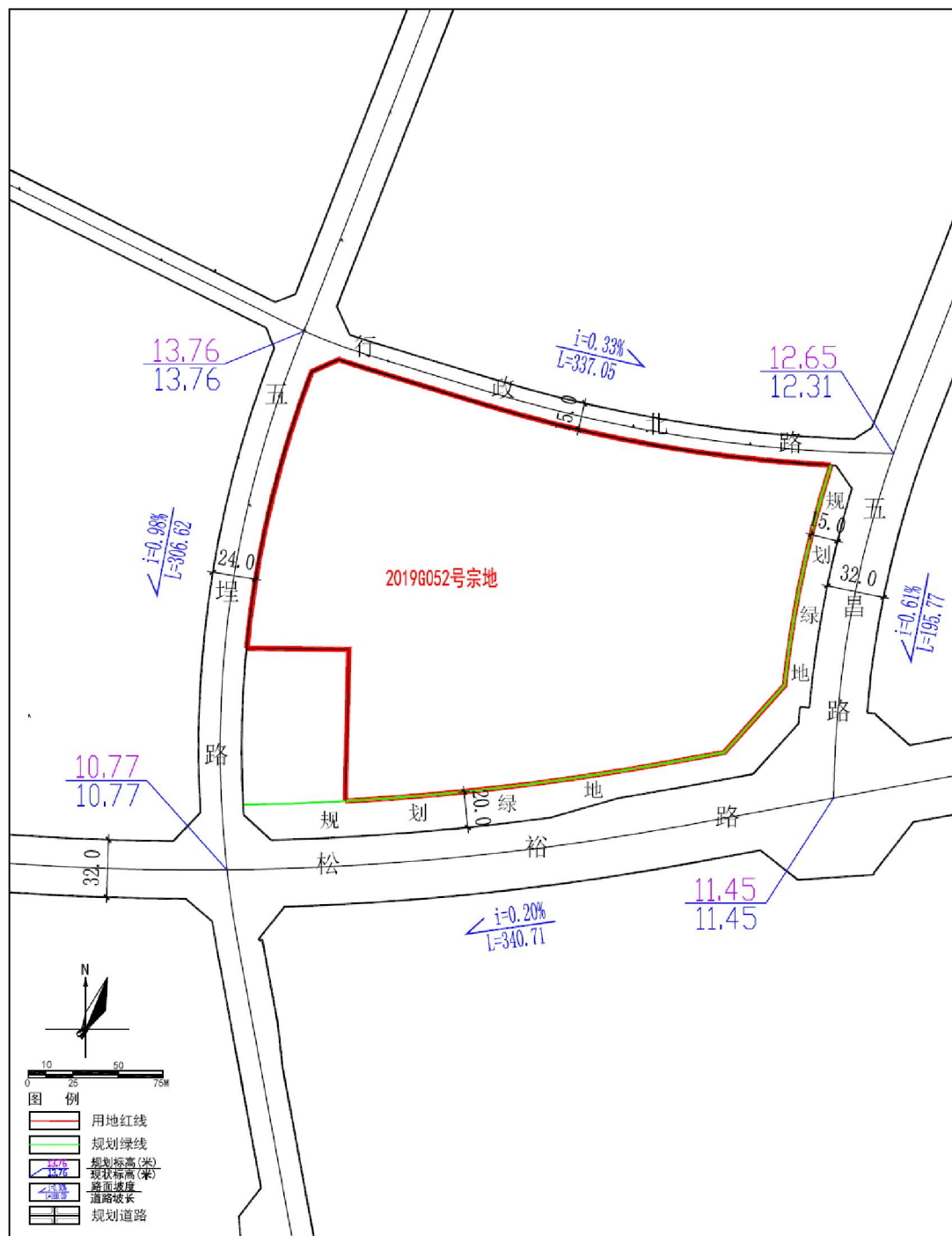
平潭综合实验区2019G052号宗地道路竖向图
