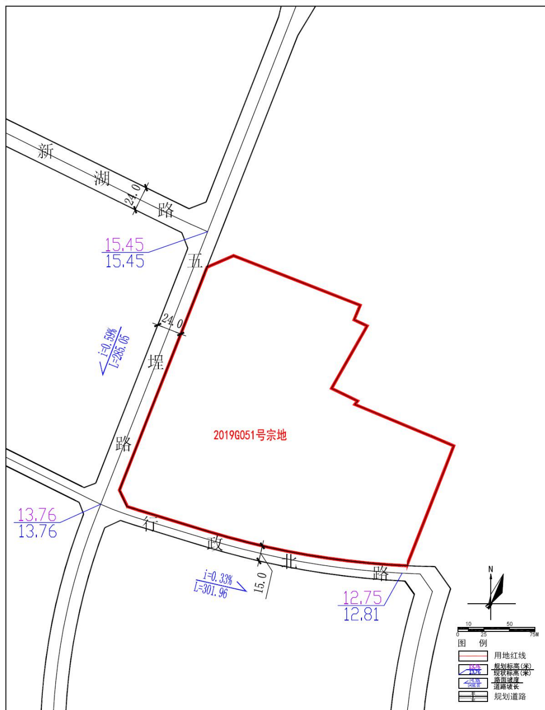
平潭综合实验区2019G051号宗地道路竖向图
