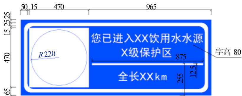
图 B.3 饮用水水源保护区道路警示牌图示及尺寸
