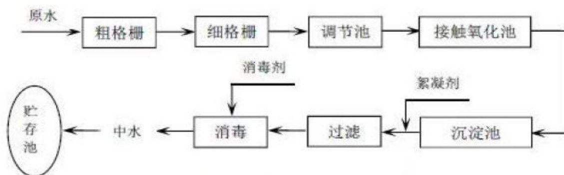
图 7.1-3 污水处理工艺流程图
