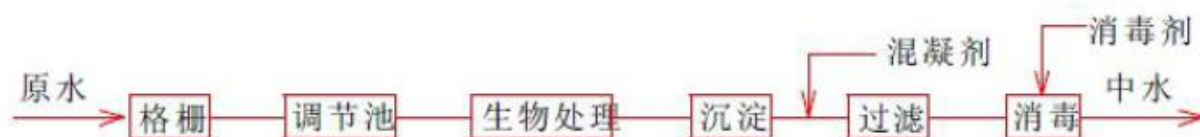
图 7.1-4 推荐污水处理基本处理工艺图
