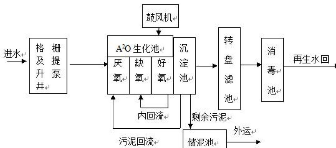
图 7.1-1 竹屿污水处理厂工艺流程图
