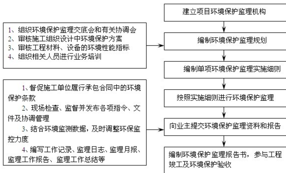
图 11-1 环境监理工作程序图
