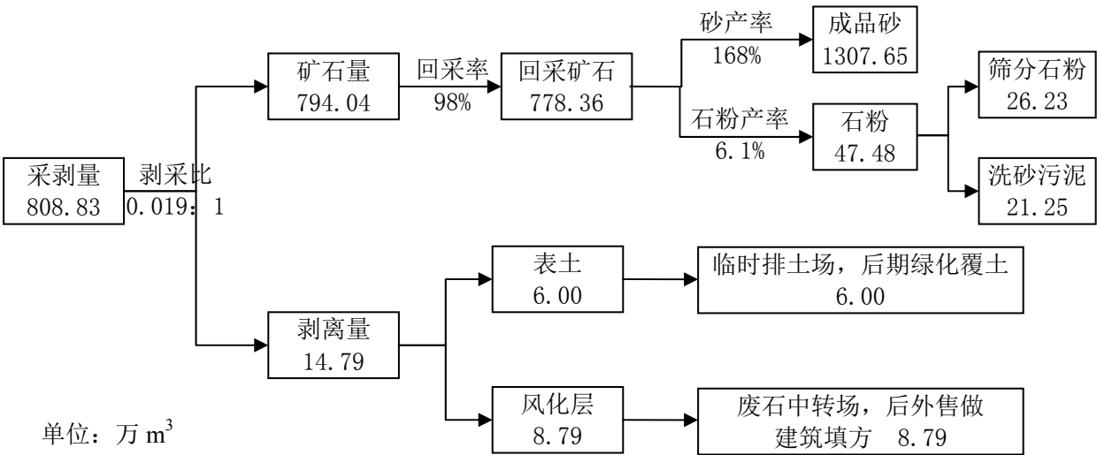
图 3-7 项目物料平衡图
