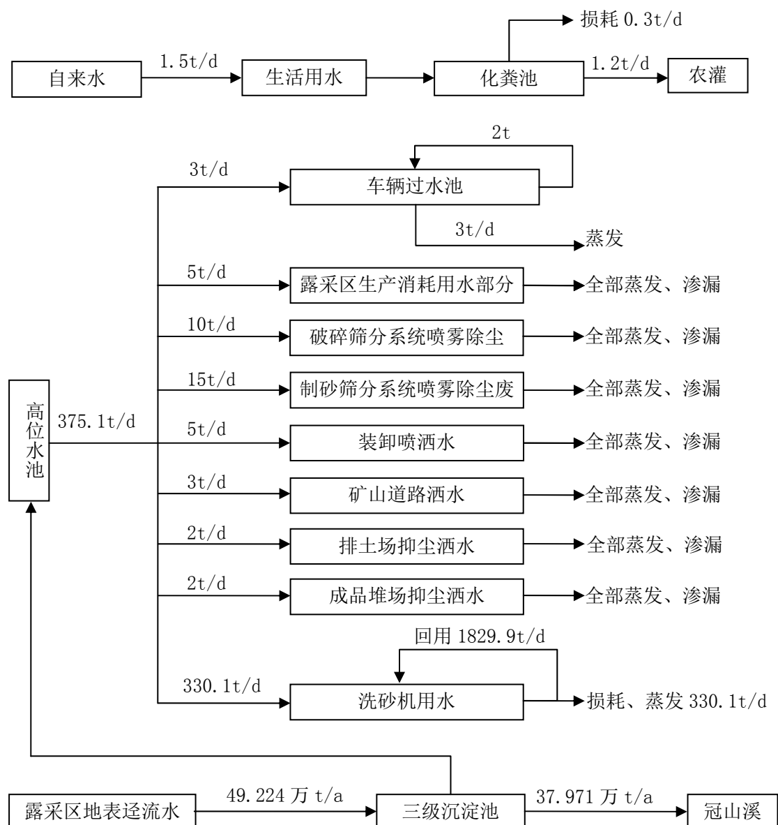
图 3-5 给排水平衡图
