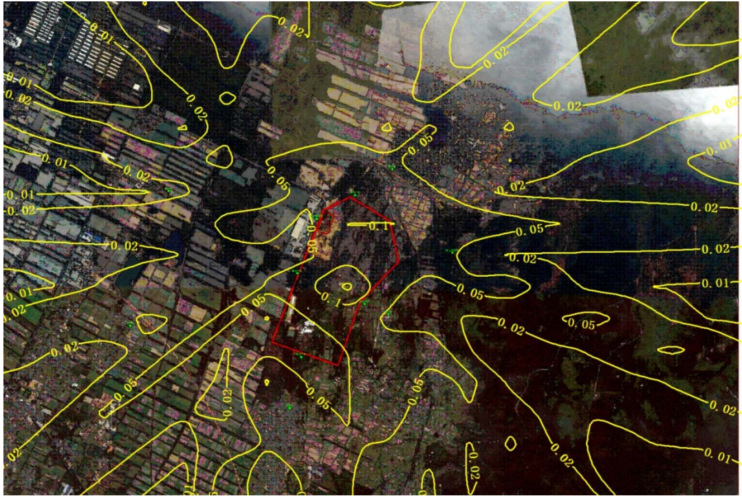
图 6-8 TSP 地面日均浓度增量分布图(单位:mg/m 3 )
