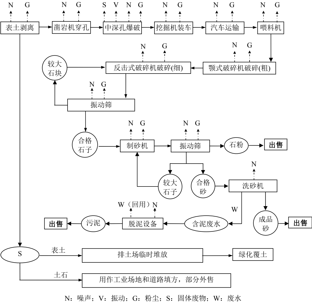
图 3-3 项目生产工艺流程及产排污环节图
