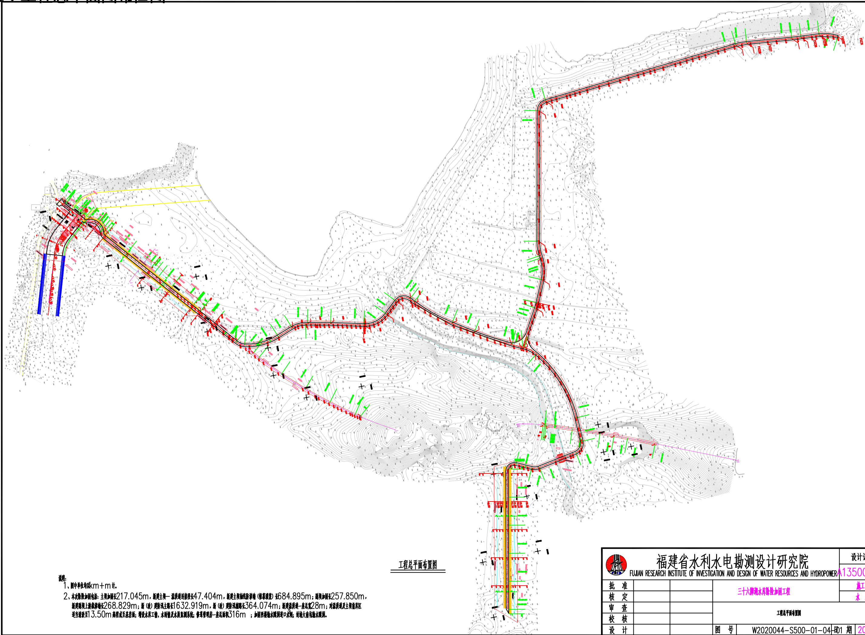
附图1：工程总平面图布置图
