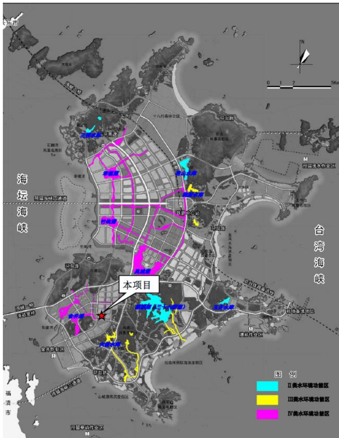
图 2.5-1 项目区水环境功能区划示意图
