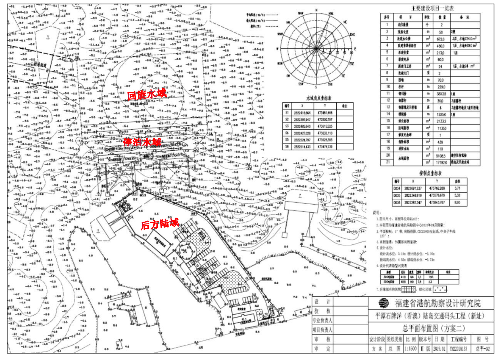
图 3.2-1 总平面布置图
