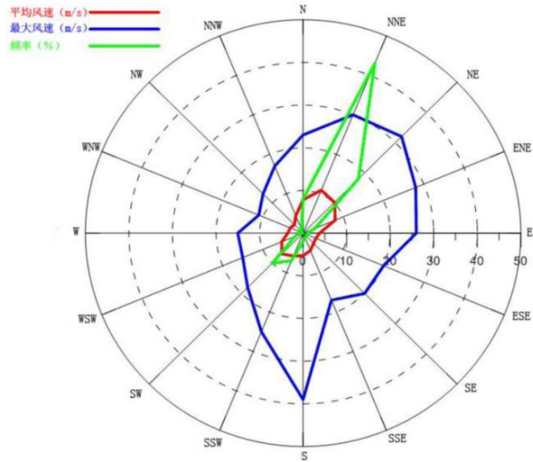
图 2.2-1 平潭海洋站风玫瑰图
