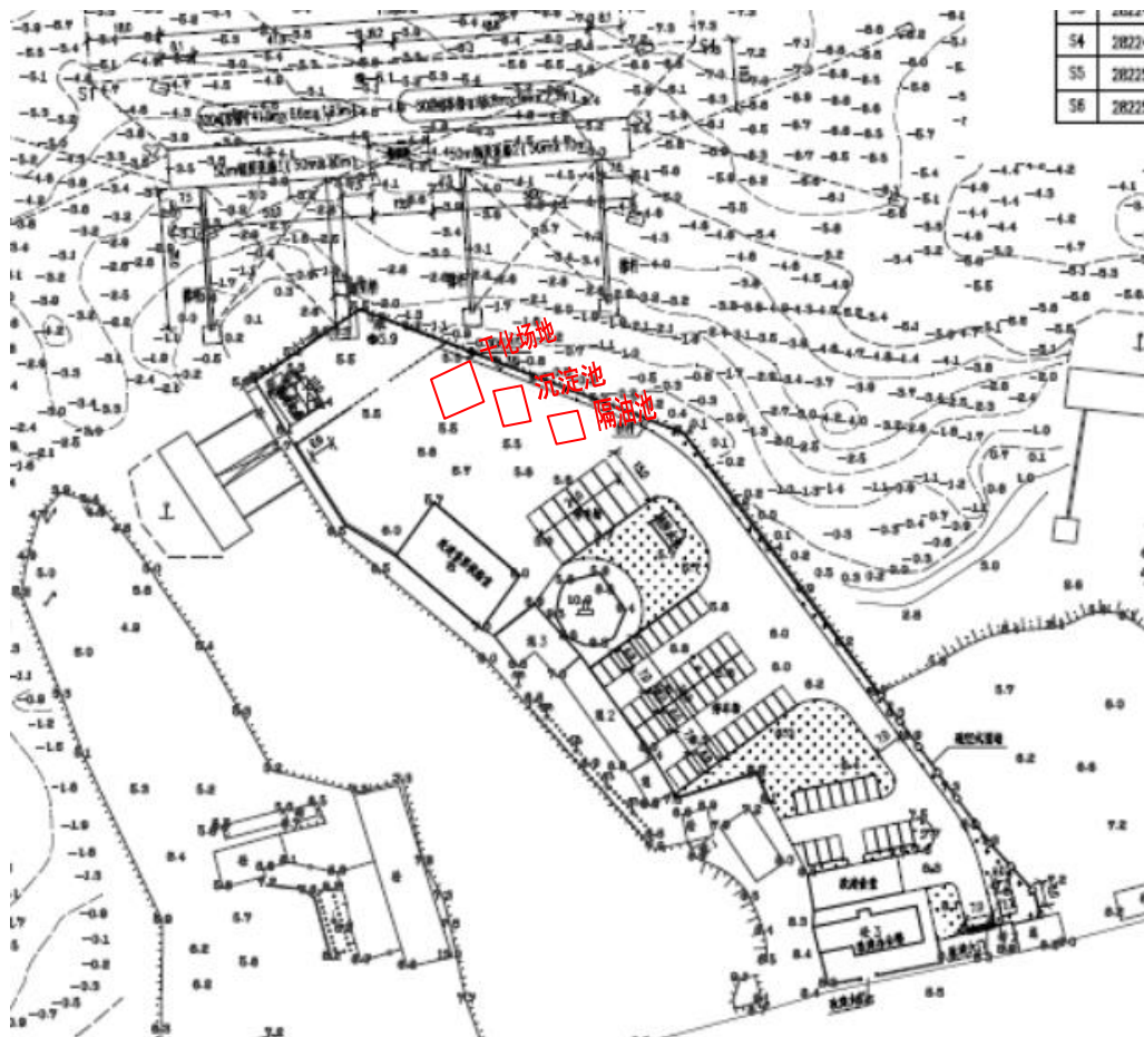
图 3.5-1 项目施工期场地平面布置示意图
