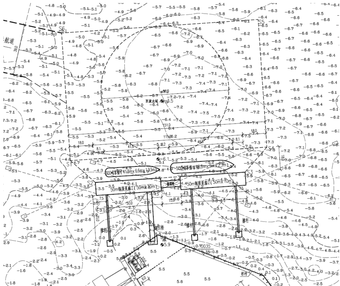
图 2.2-3 水深地形图
