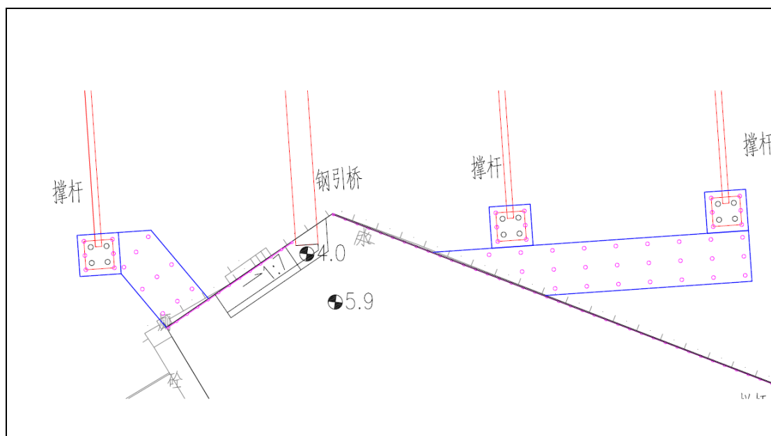
图 3.5-2 工作平台布置情况
