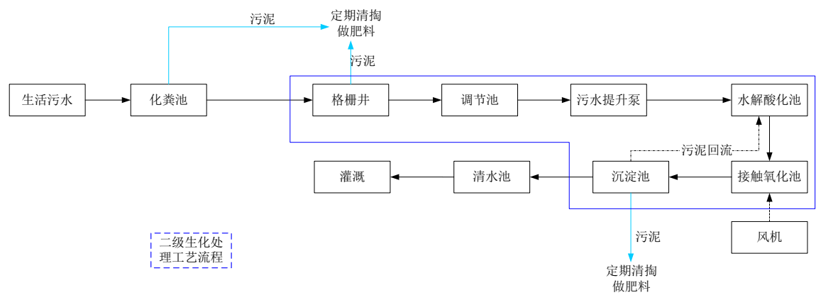
图 5.2-2 污水处理工艺流程
