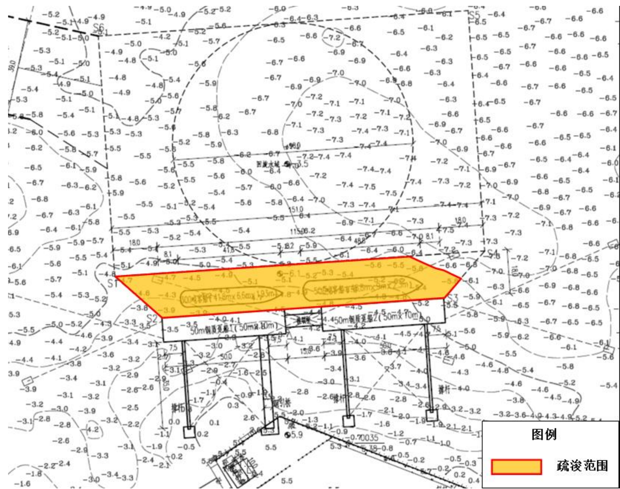
图 3.2-2 疏浚工程平面布置图
