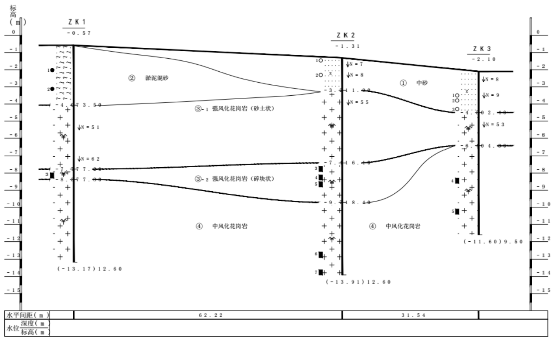
图 2.2-5 地质剖面 1-1'
