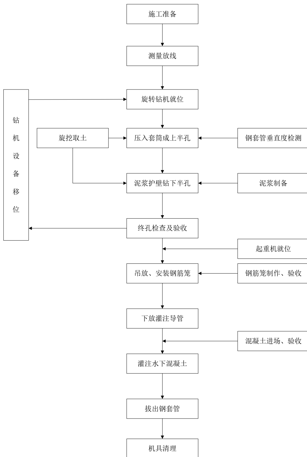
图 3.5-3 灌注桩施工流程图
