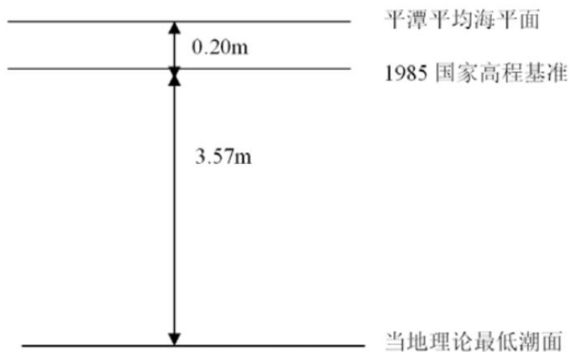
图 2.2-2 平潭海域各高程基准面换算关系图
