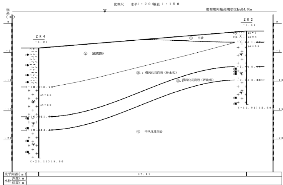
图 2.2-6 地质剖面 2-2'
