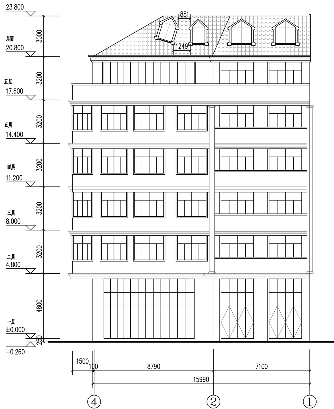
④~①轴立面图 1:120
