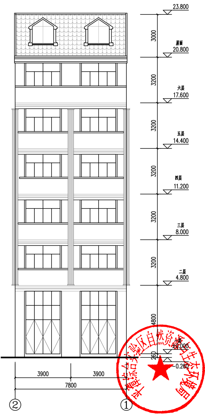
②~①轴立面图 1:120
