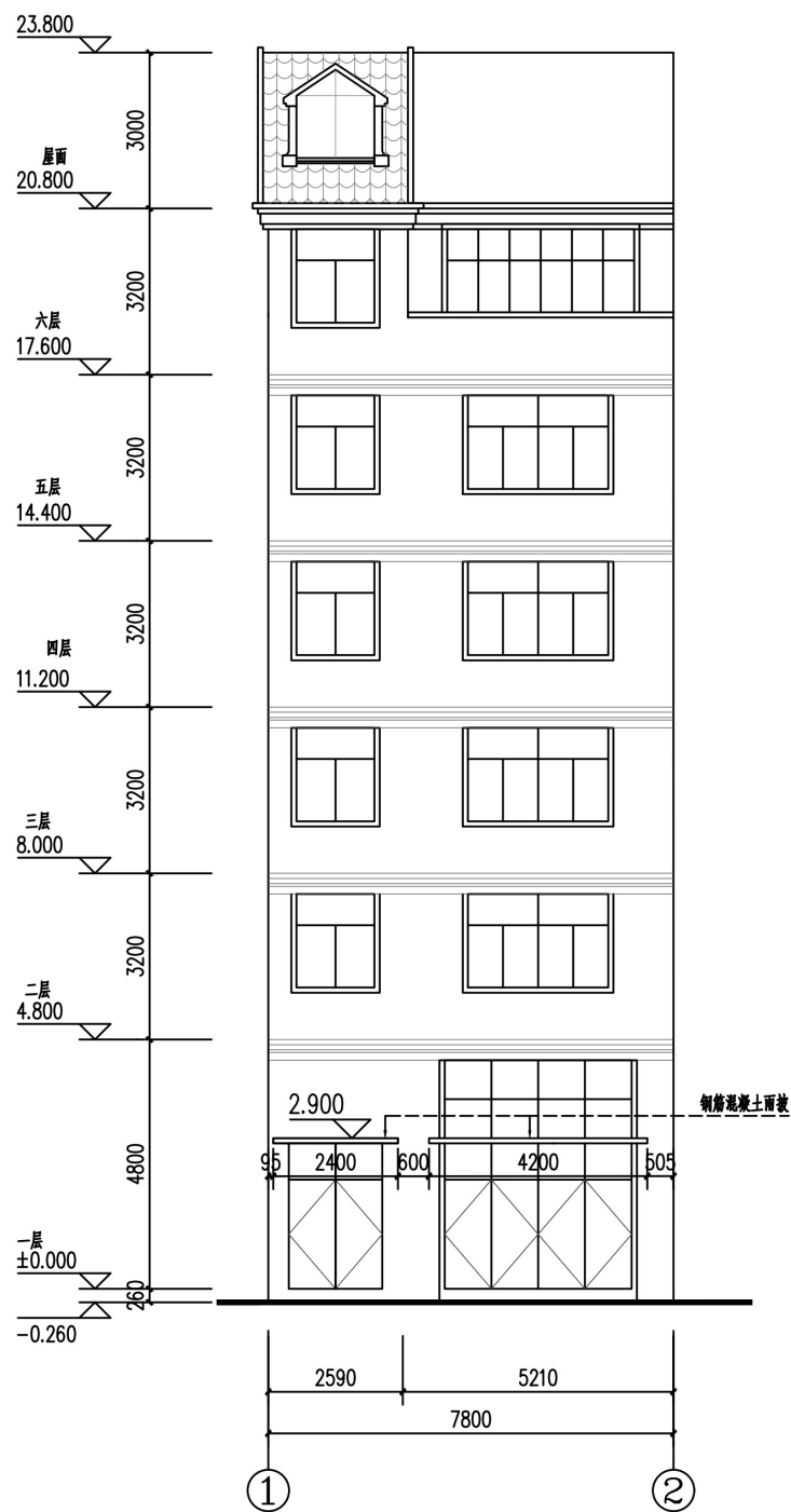
①~②轴立面图 1:120
