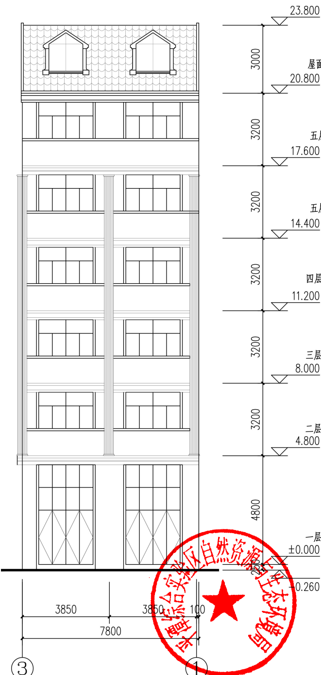
③~①轴立面图 1:120 北立面·沿街立面
