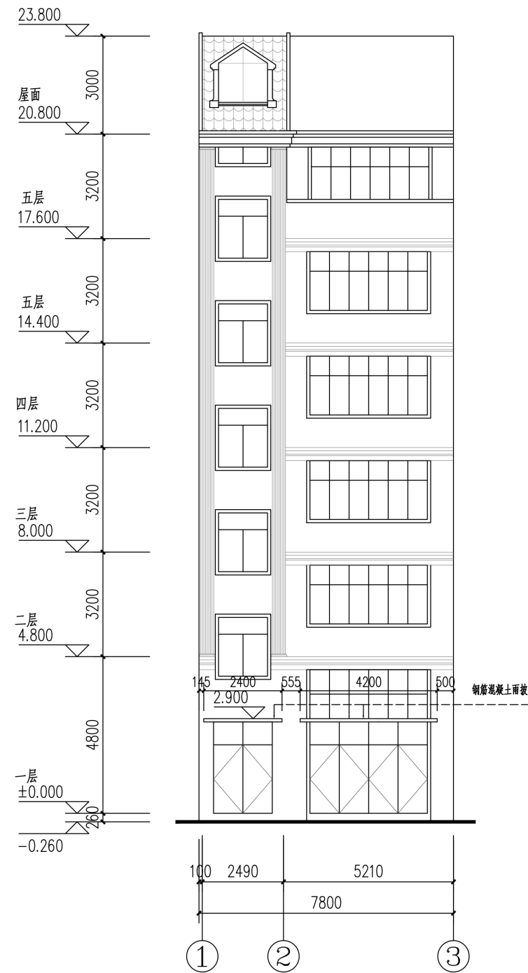
①~③轴立面图 1:120 南立面
