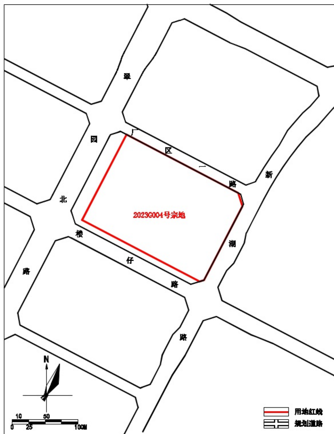
平潭综合实验区2023G004号宗地位置图
