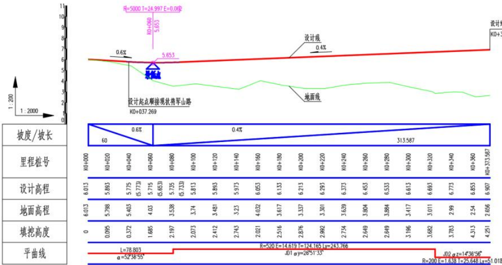
图2-3 道路纵断面图
