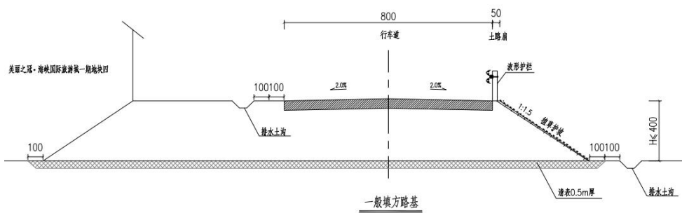
图2-6 一般填方路基图
