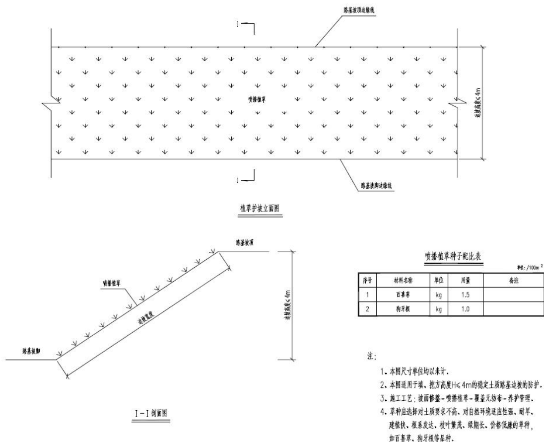
图 4-1 道路生态保护典型措施设计图
