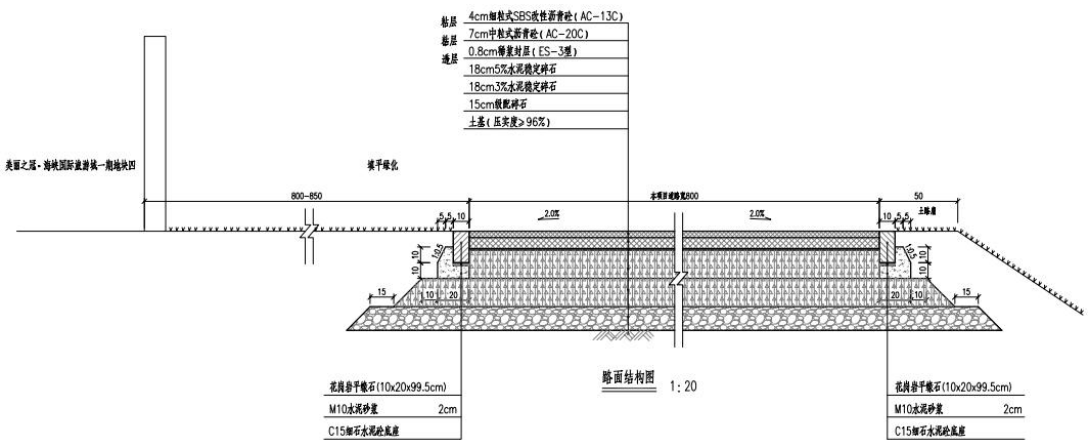
图2-5 路面结构图
