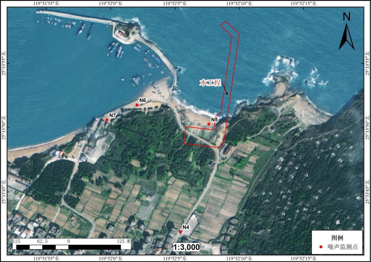
附图 13 噪声监测站位图
