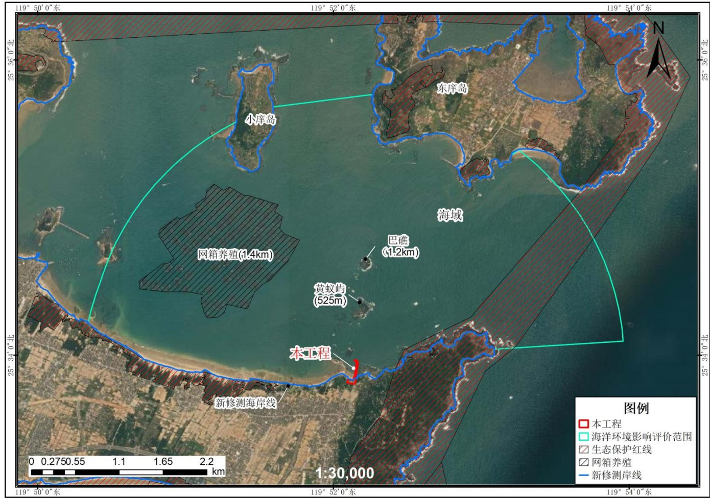
附图 14 生态环境保护目标图（海洋）
