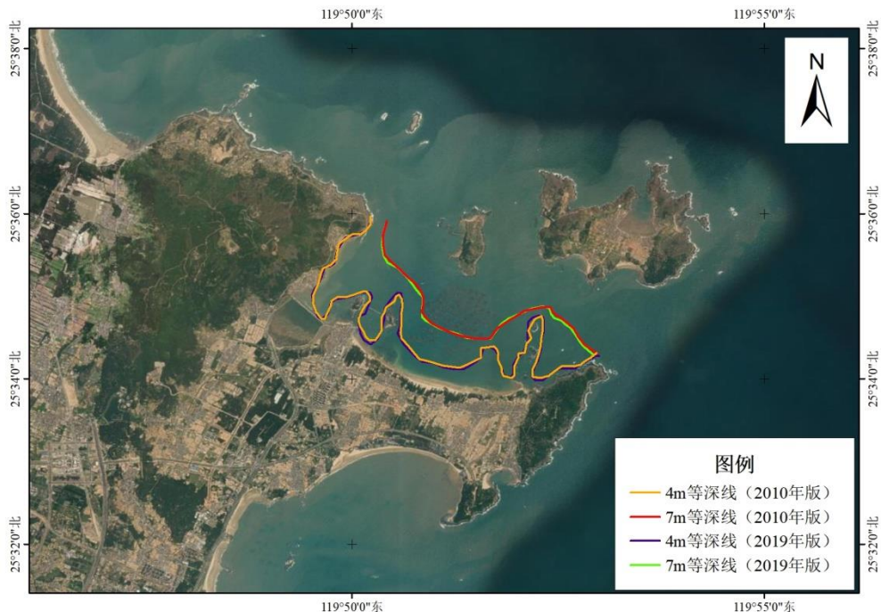
图 3-4 2010 年版与 2019 年版海图等深线对比
