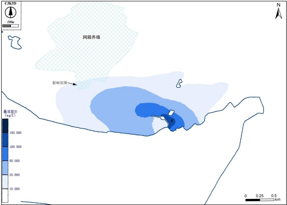
图 4-2 施工期悬浮物全潮最大影响包络范围图
