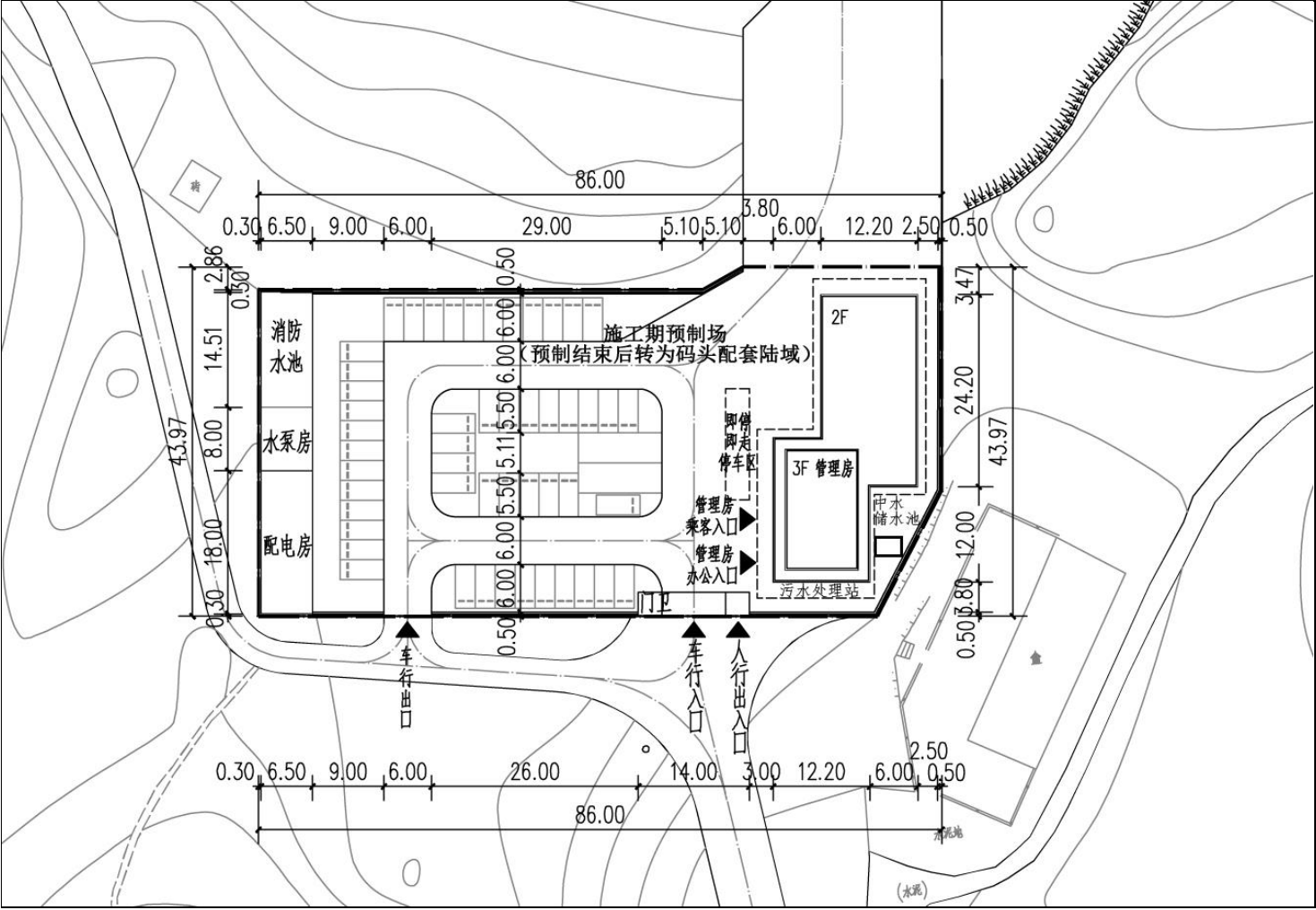
附图 3 总平面布置图（陆域）
