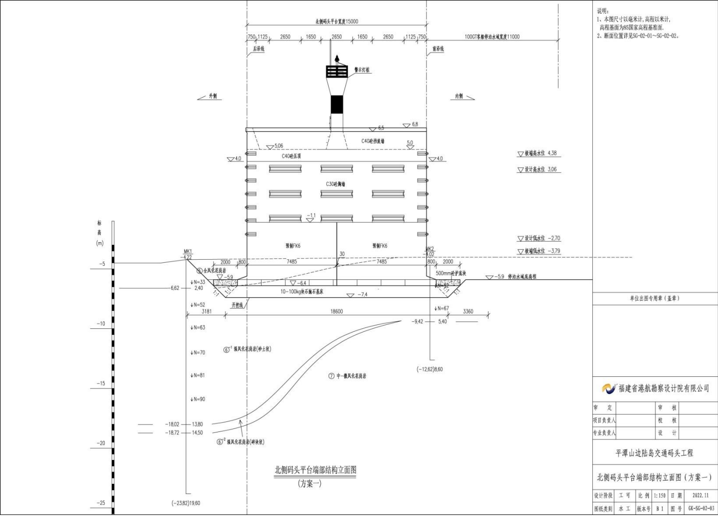
附图 5 北侧码头平台端部结构立面图
