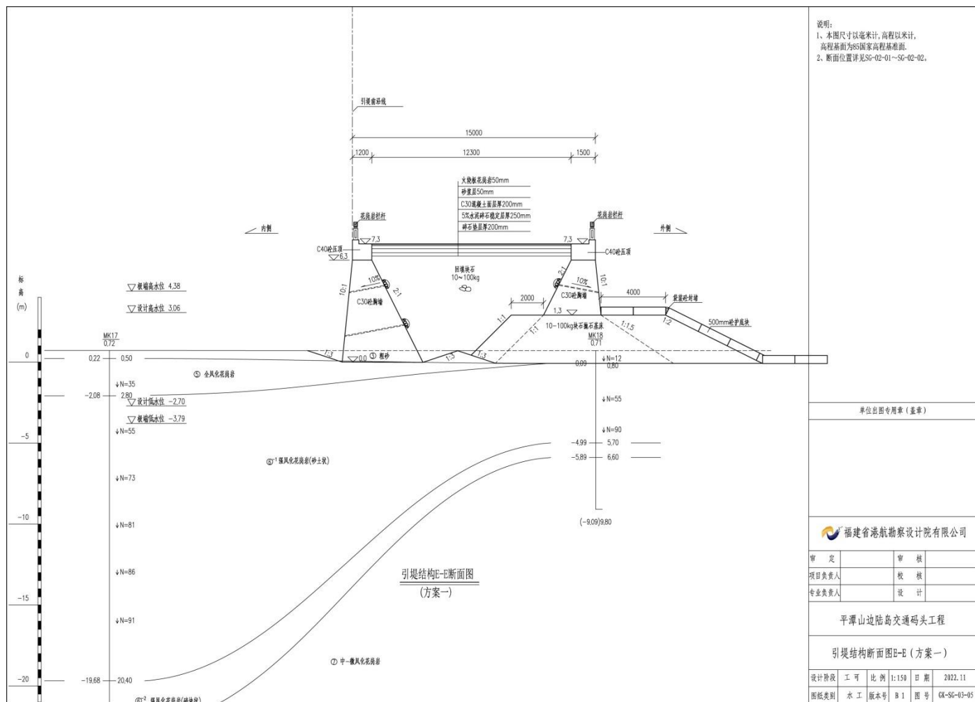
附图 7 码头结构断面图 (引堤 E-E 断面)
