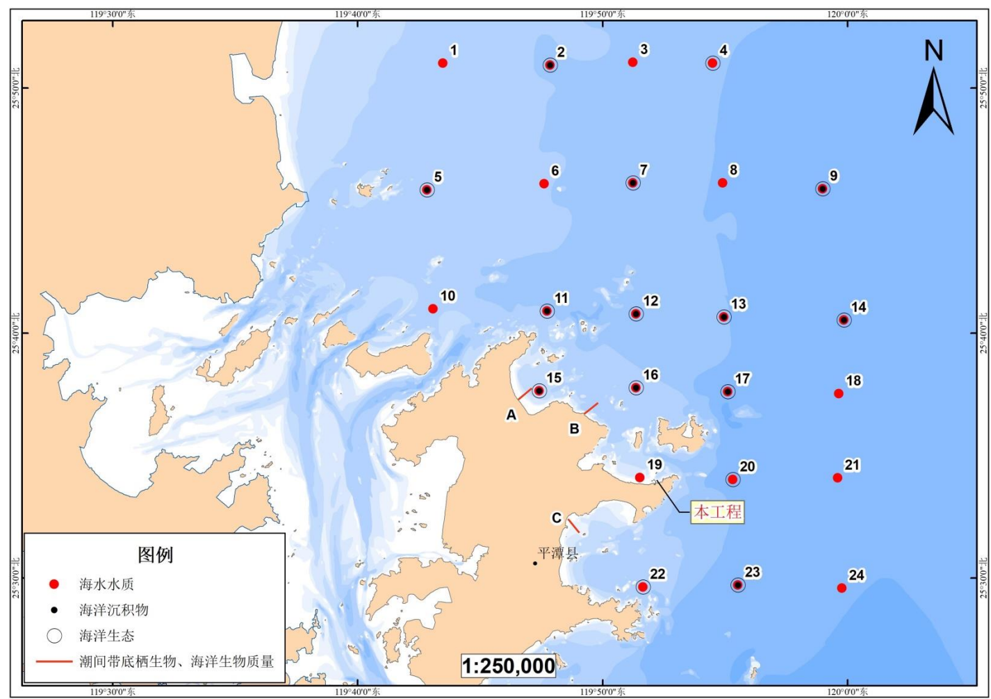
附图 12 项目周边海域海洋环境现状调查站位图（2022 年 11 月）
