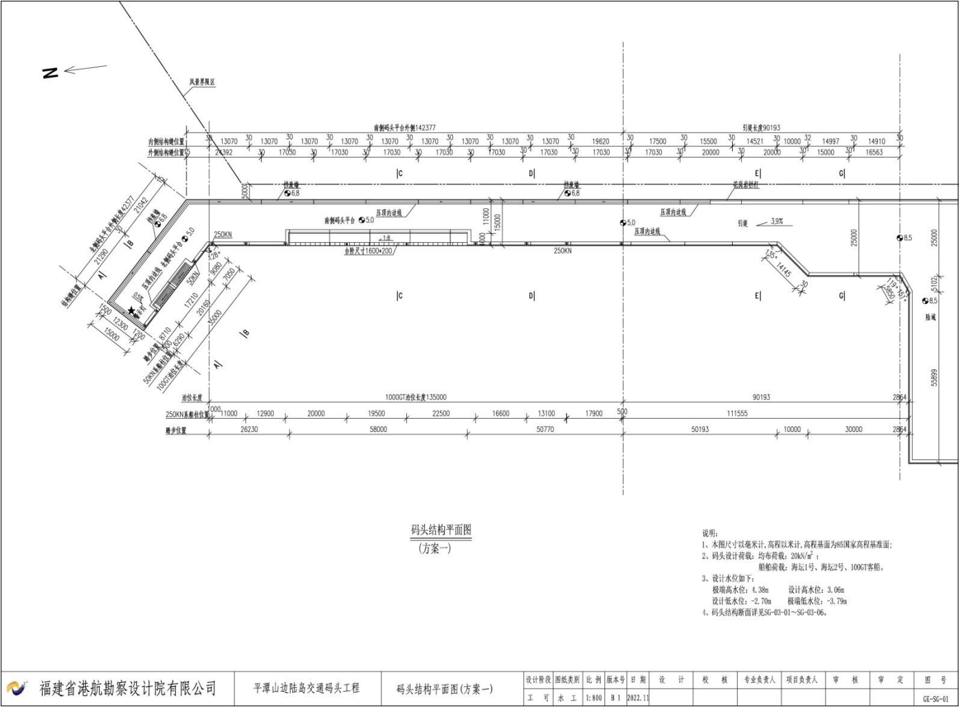
附图 4 码头结构平面图
