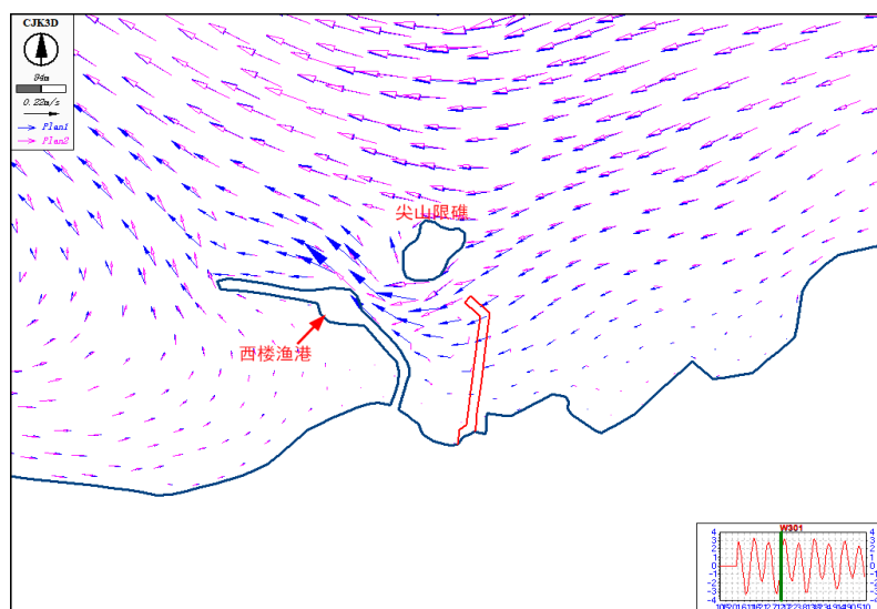
图 4-8 工程前后大潮涨急时刻流场对比图
