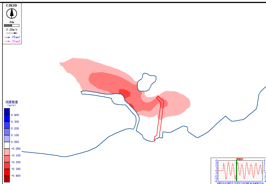
图 4-11 工程前后大潮期工程附近涨急时刻流速变化分布图
