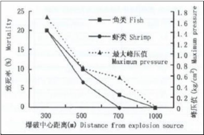
图 4-3 爆破对生物的致死率与爆破中心的距离关系
