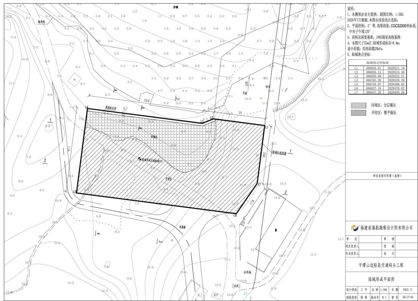
附图 8 陆域形成平面图
