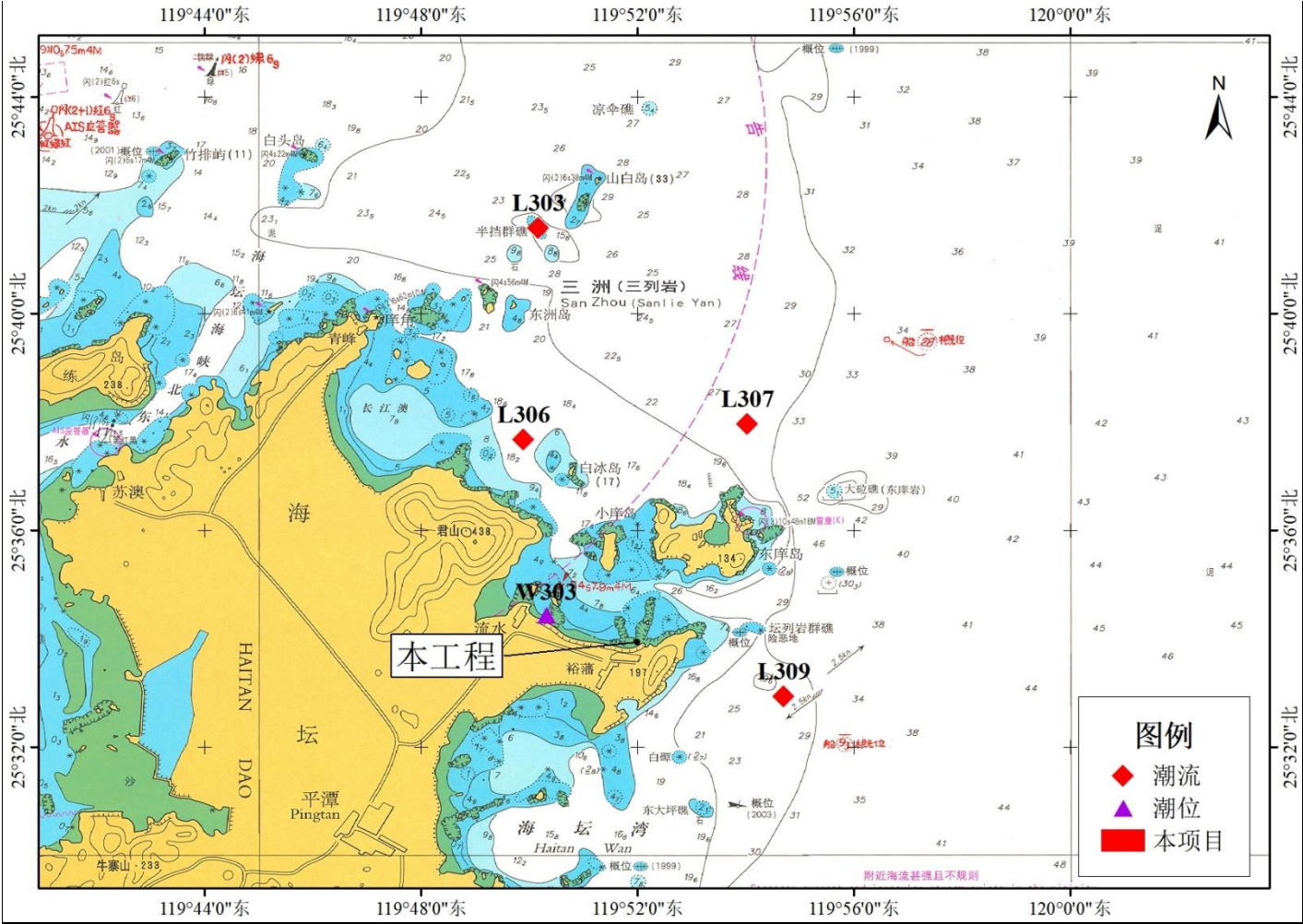
附图 11 项目周边海域水文监测站位图
