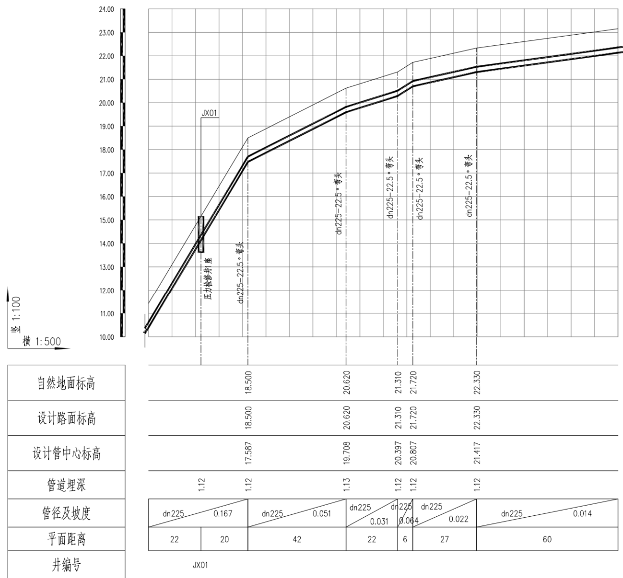
附图 4.2 本项目管道纵断面图
