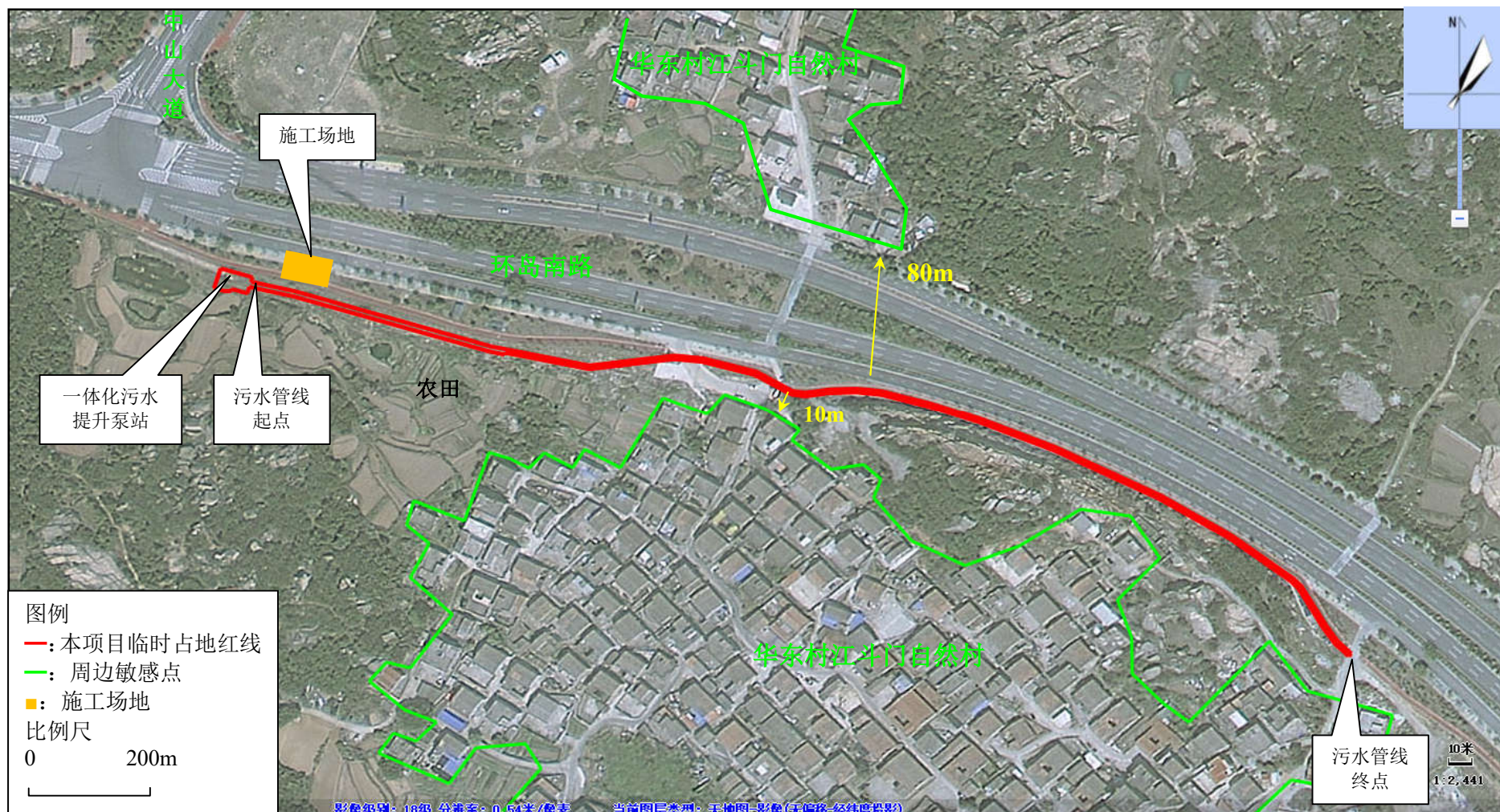
附图2 项目总体布局及周边敏感目标分布图
