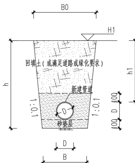
图 2-2 管道敷设及土石方回填形式图
