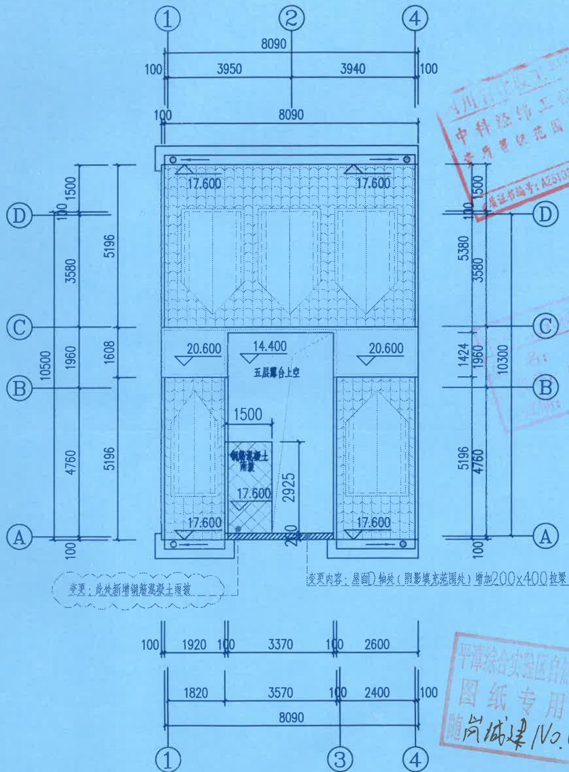
屋面平面图 (变更后) 1:100
