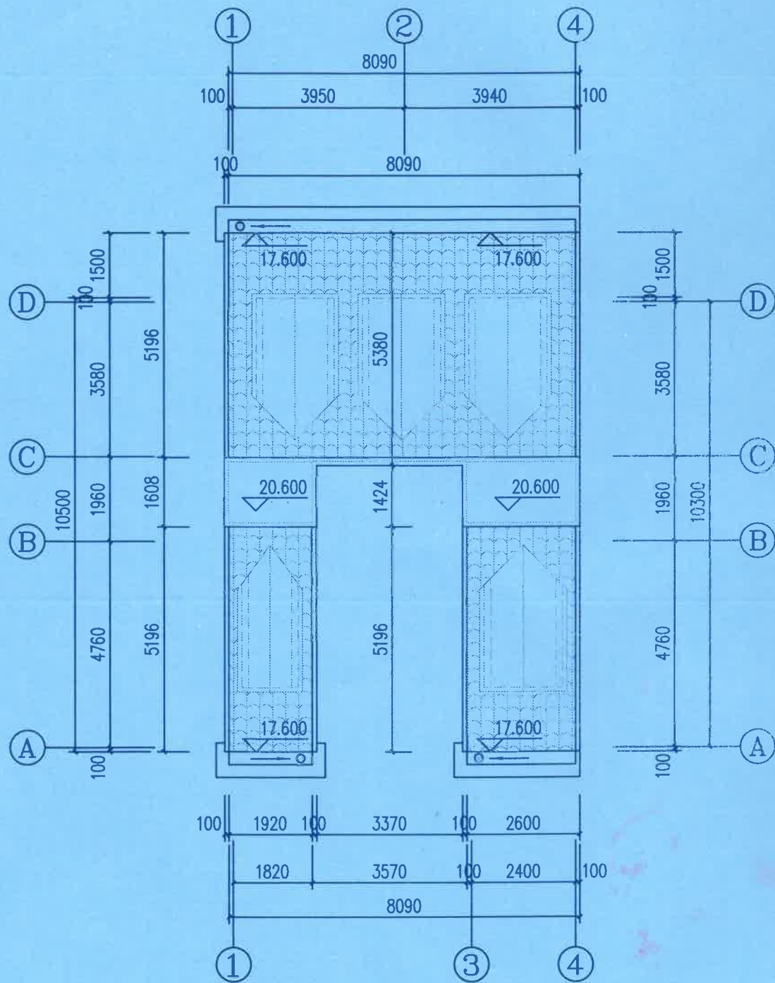
屋面平面图 (变更前) 1:100
