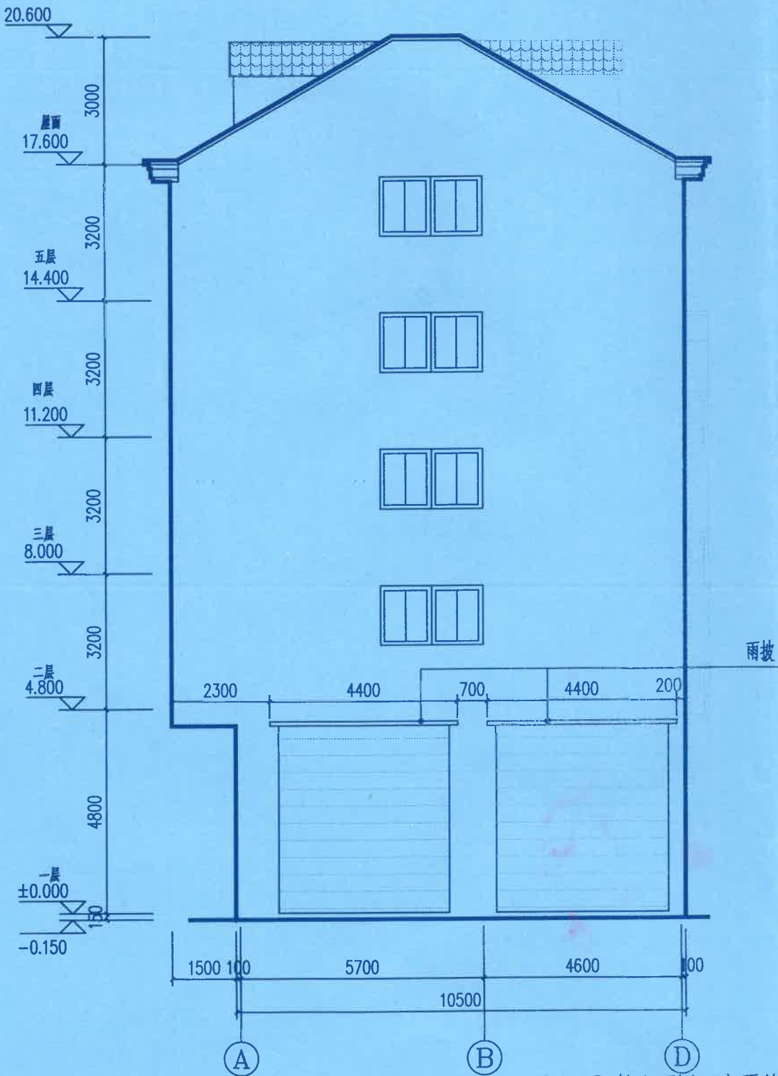
(A)~(D)轴立面图 (变更前) 1:100
