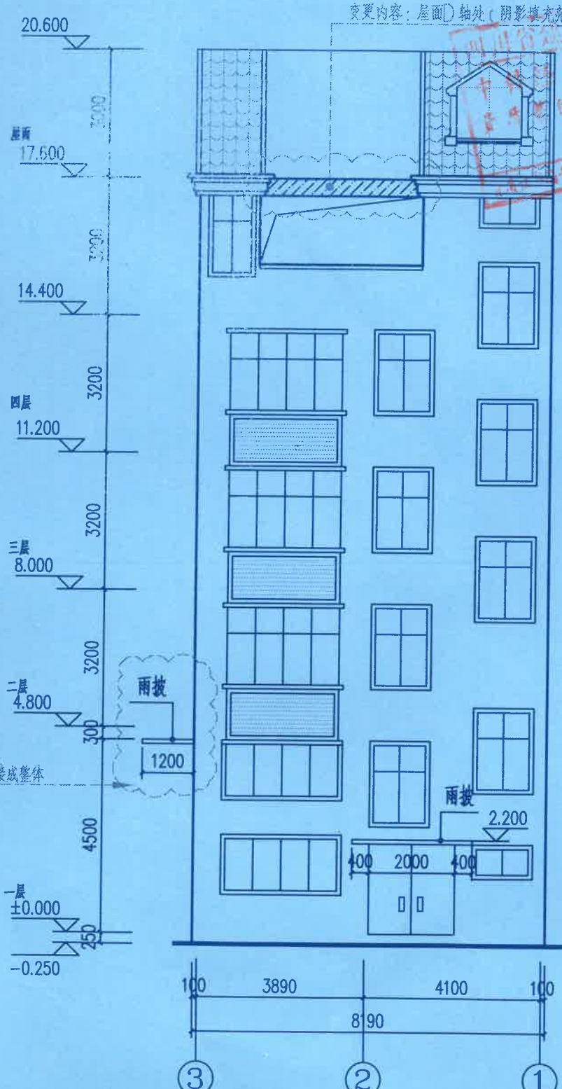
③~①轴立面图 (变更后) 1:100 (北立面)
