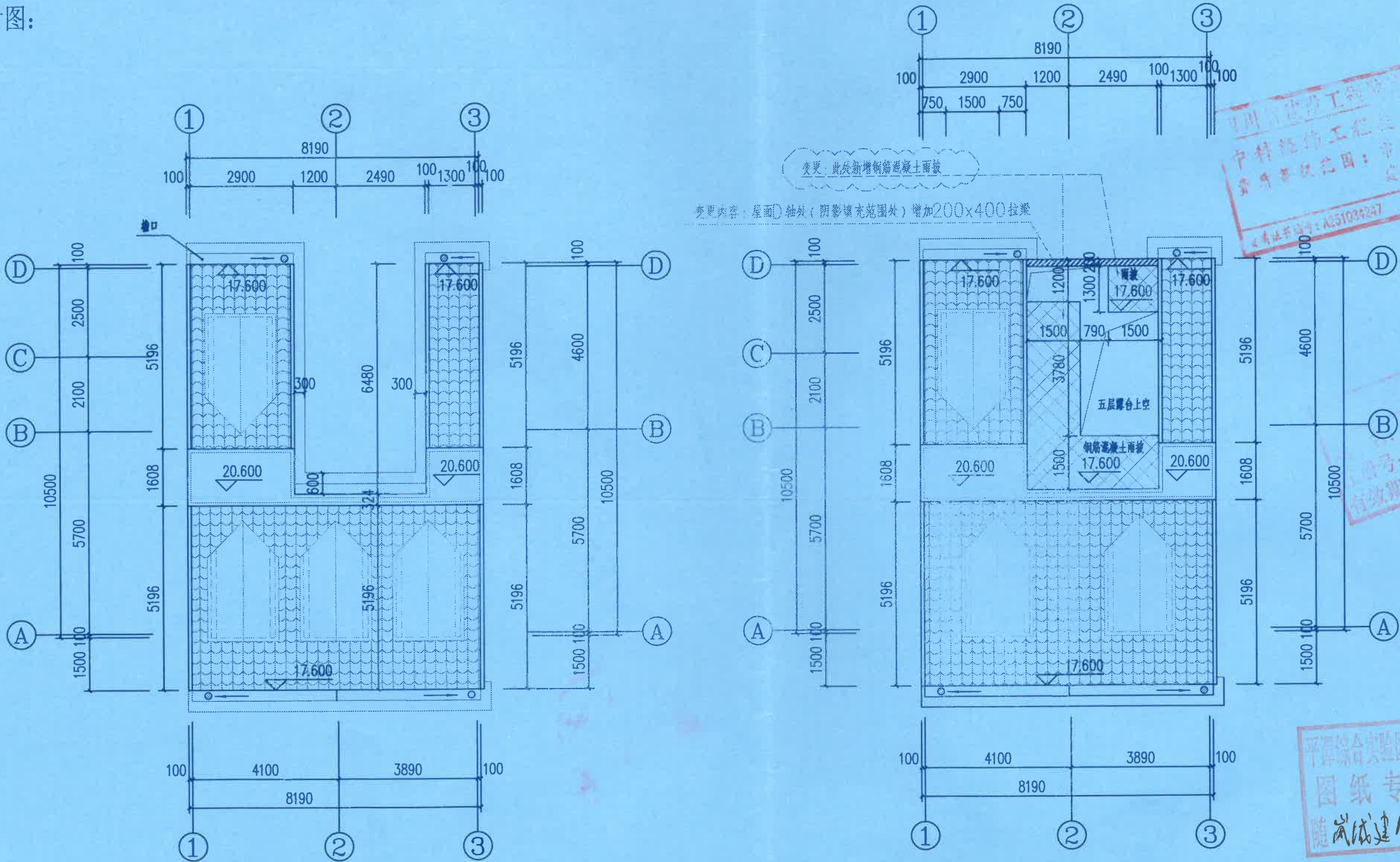
屋面平面图（变更前）1:100
