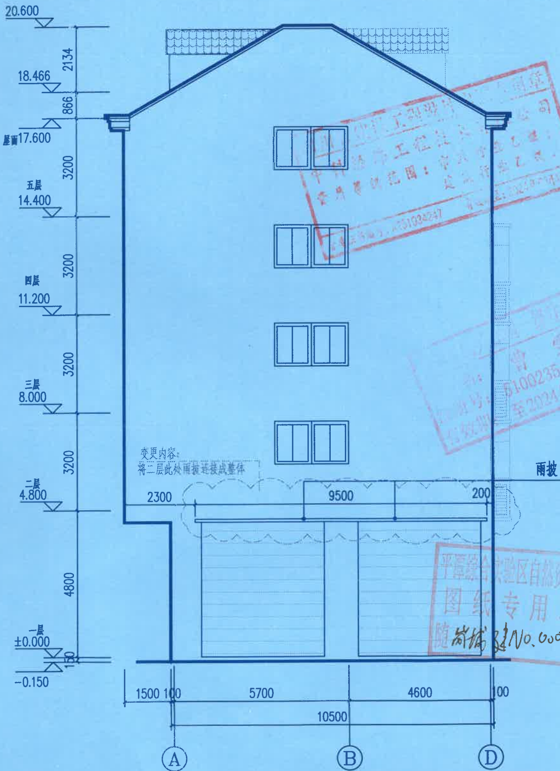
(A)~(D)轴立面图 (变更后) 1:100
