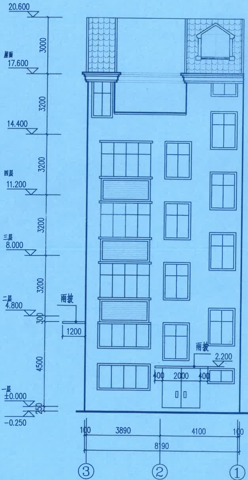
③~①轴立面图 (变更前) 1:100 (北立面)
