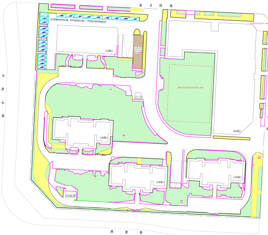
台胞社区调整后总图（地面车位及绿地）
