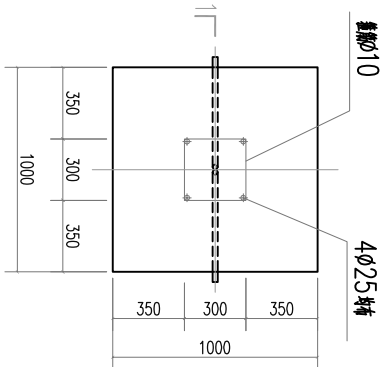
基础平面图
