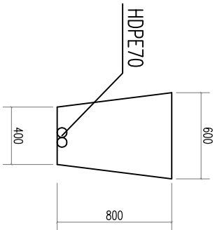
埋设电缆保护管断面
