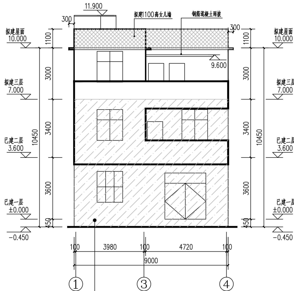
1~4 轴加层后立面图 1:100 (正立面图·南立面)
