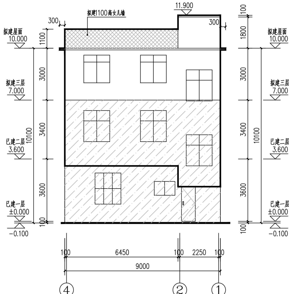
4~1 轴加层后立面图 1:100 (背立面图·北立面)
